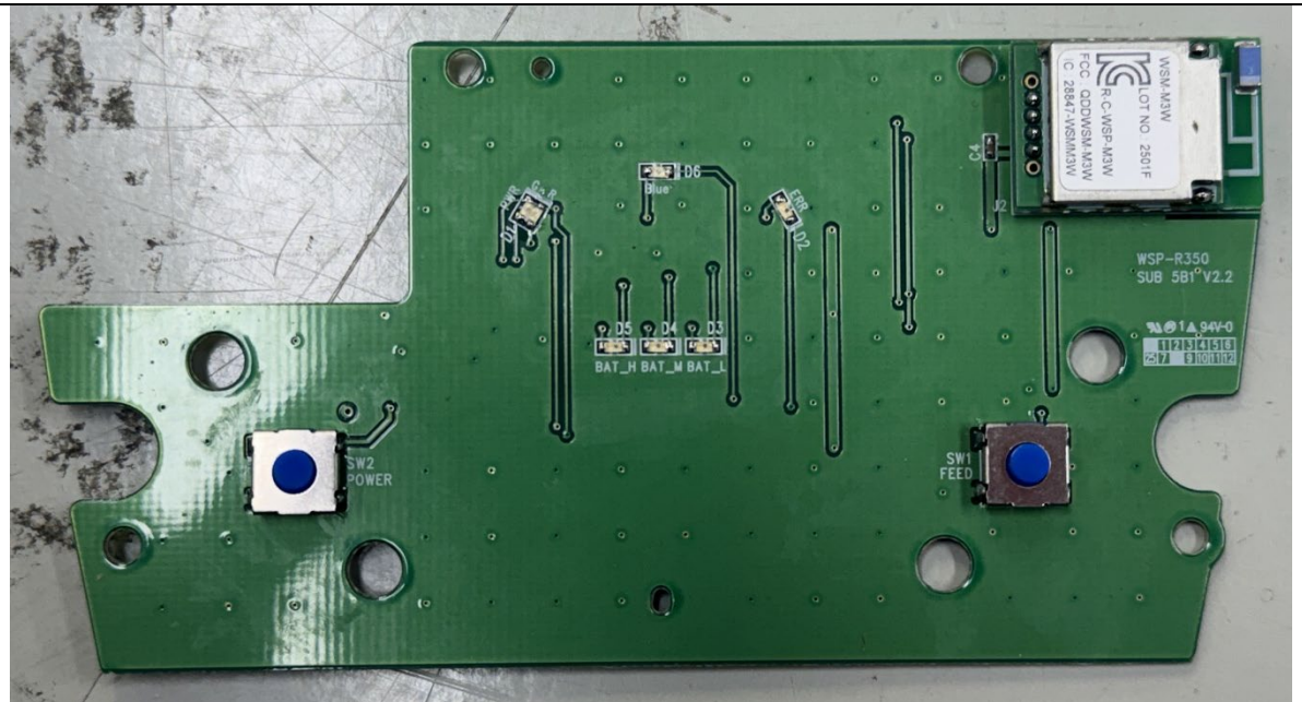
(SUB PCB_Front)
