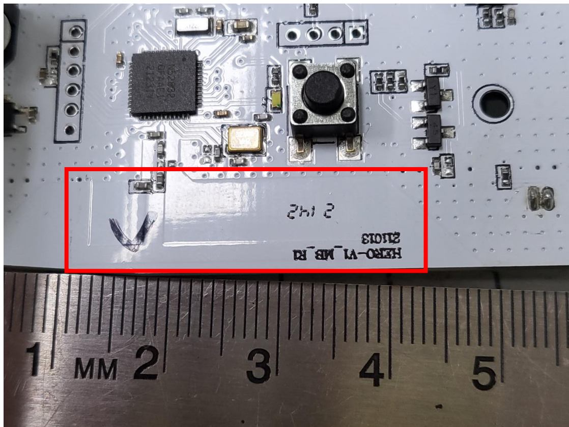
Antenna
