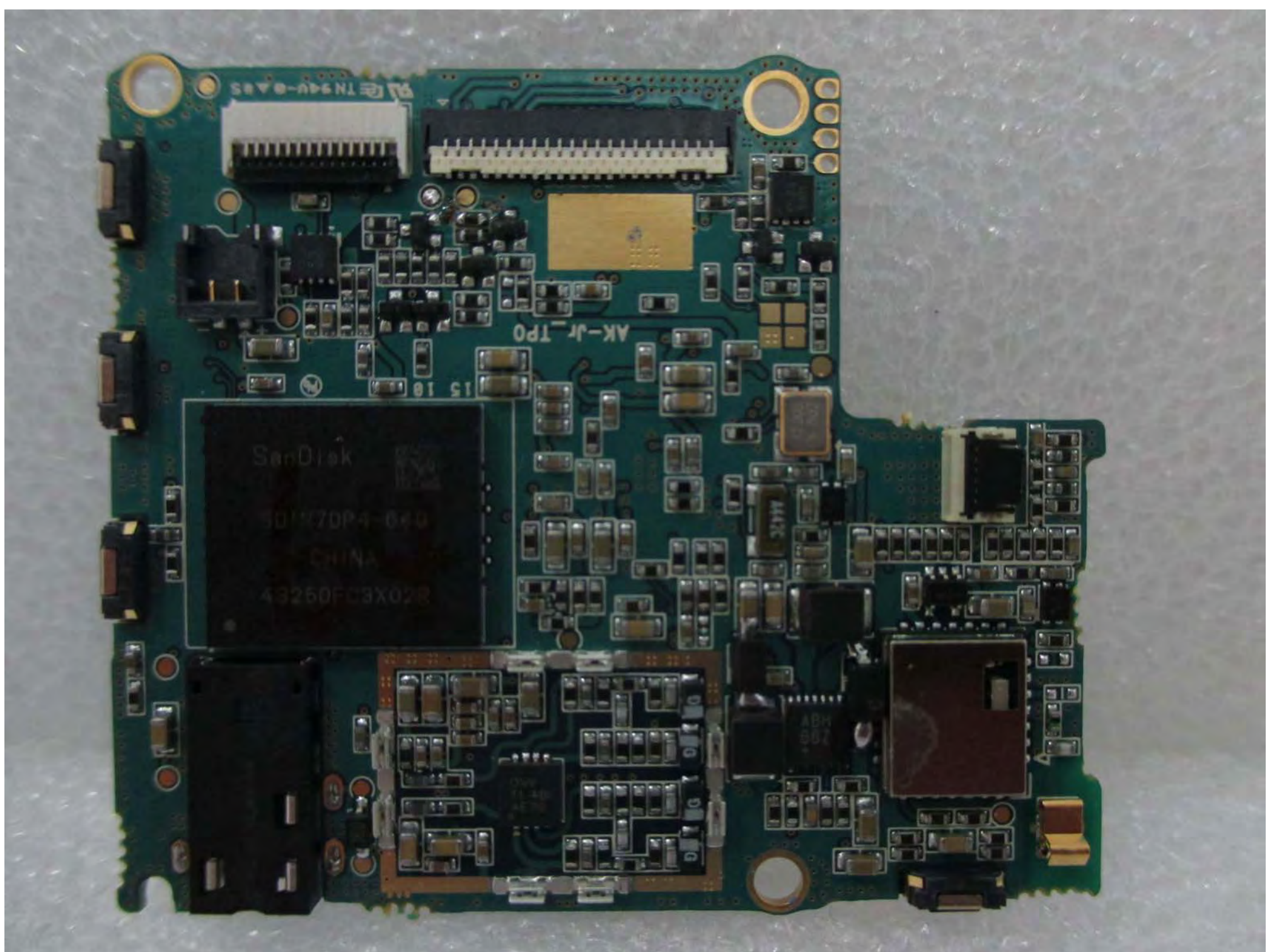
PPE11_메인보드 후면
