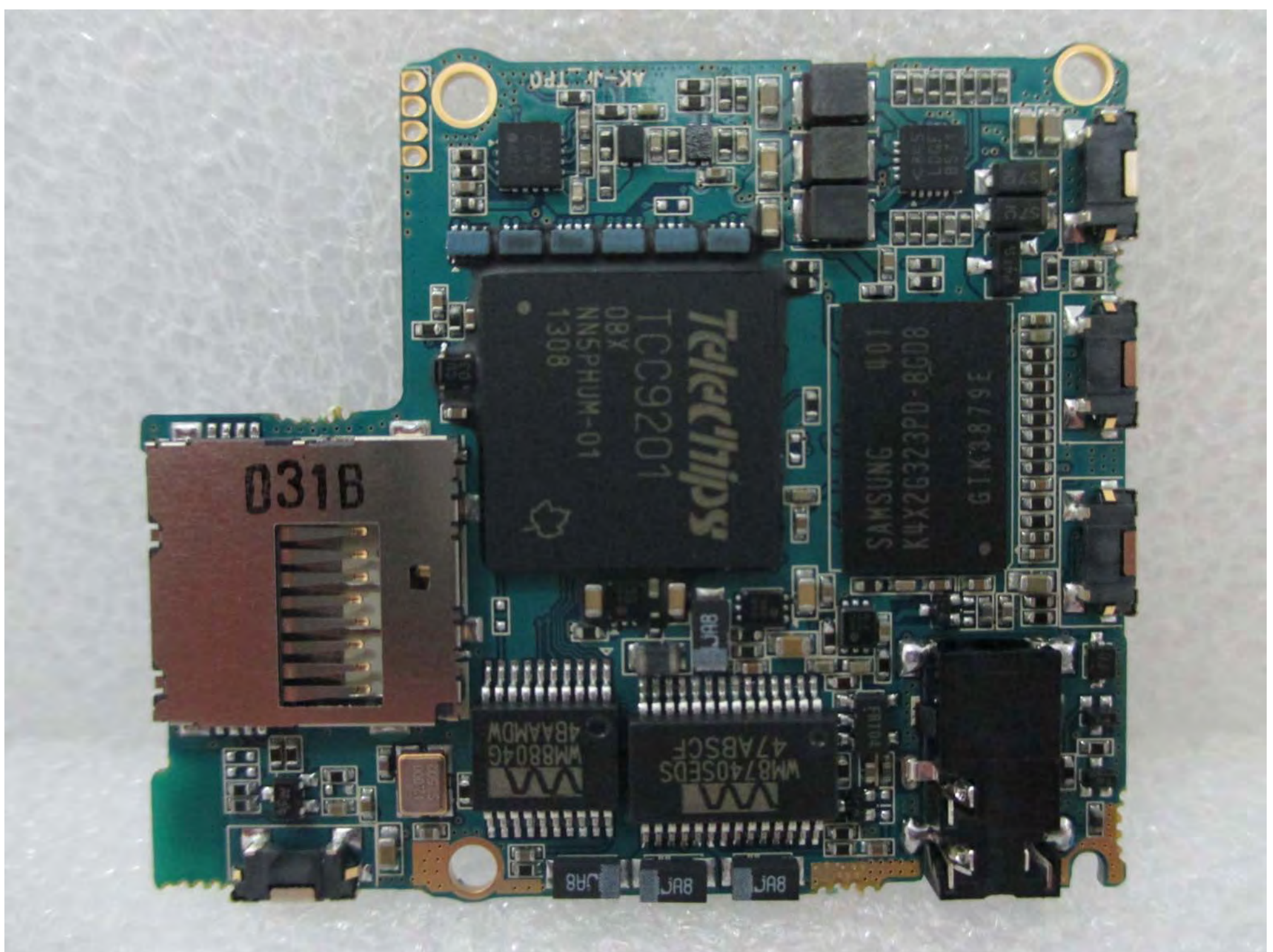
PPE11_메인보드 전면
