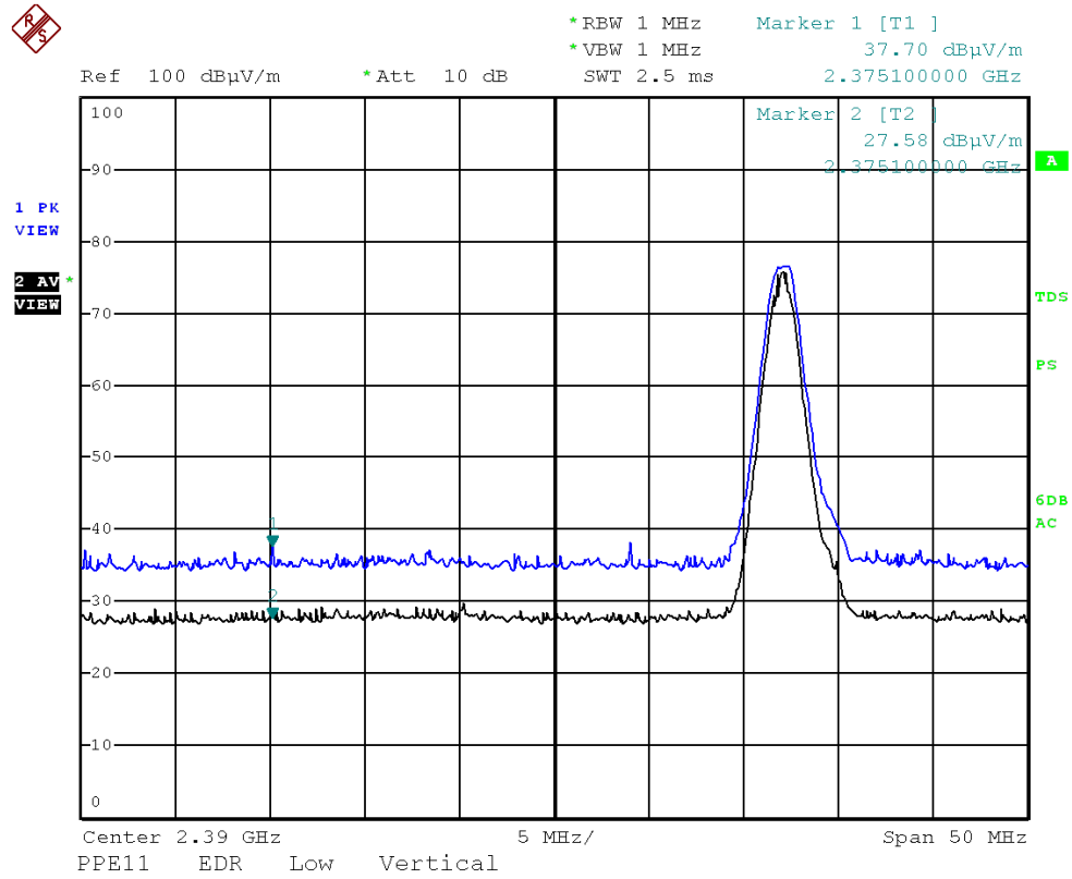
EDR(3DH5) Low(Vertical)
