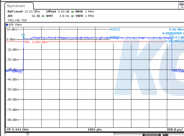
3-DH5
