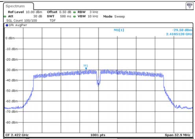
802.11n_HT40 / 2 422 MHz
