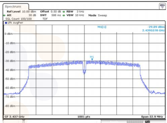
802.11n_HT40 / 2 437 MHz
