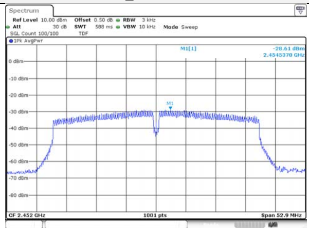
802.11n_HT40 / 2 452 MHz
