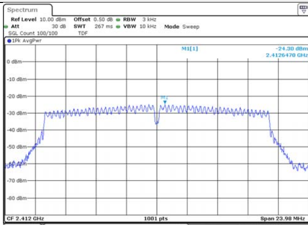
802.11n_HT20 / 2 412 MHz
