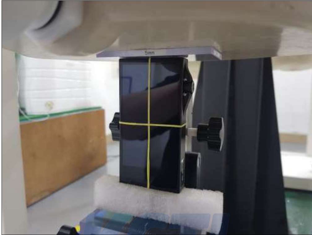
Top (5 mm)
