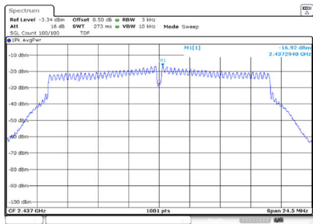
802.11n_HT20 / 2 437 MHz
