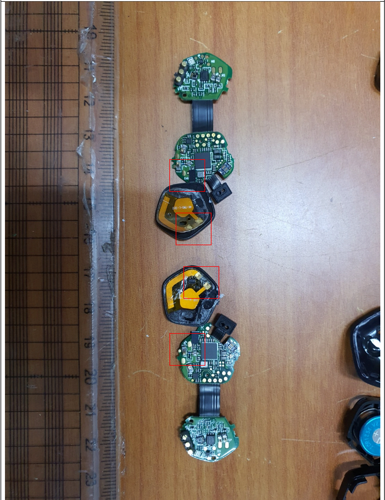
ANTENNA(2.4 GHz)
