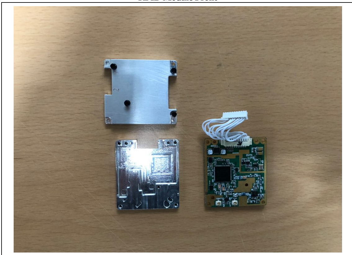
RFID Module Front
