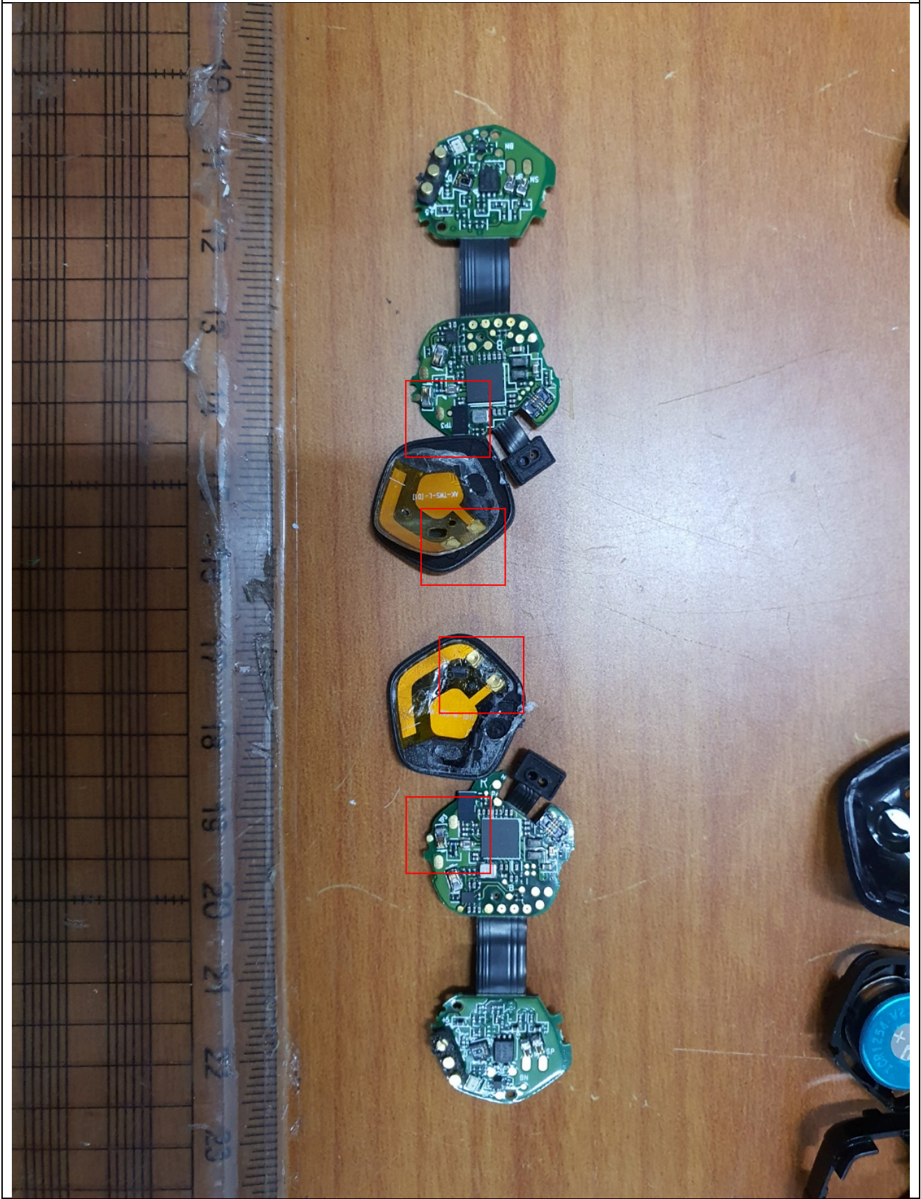
ANTENNA(2.4 GHz)
