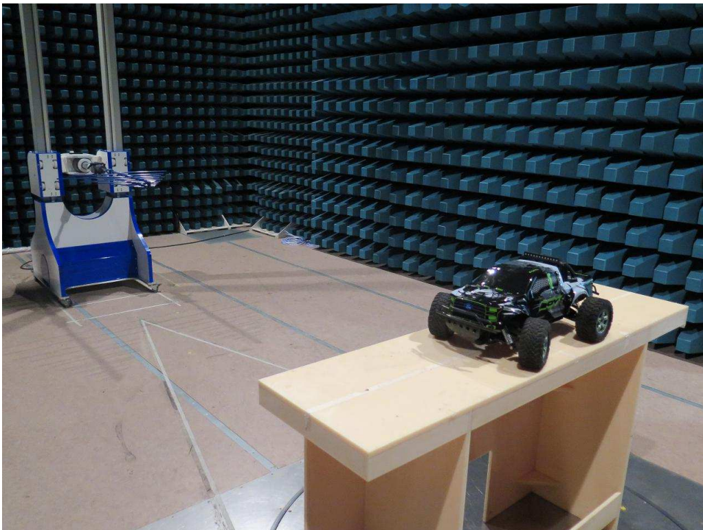
300MHz – 1GHz
