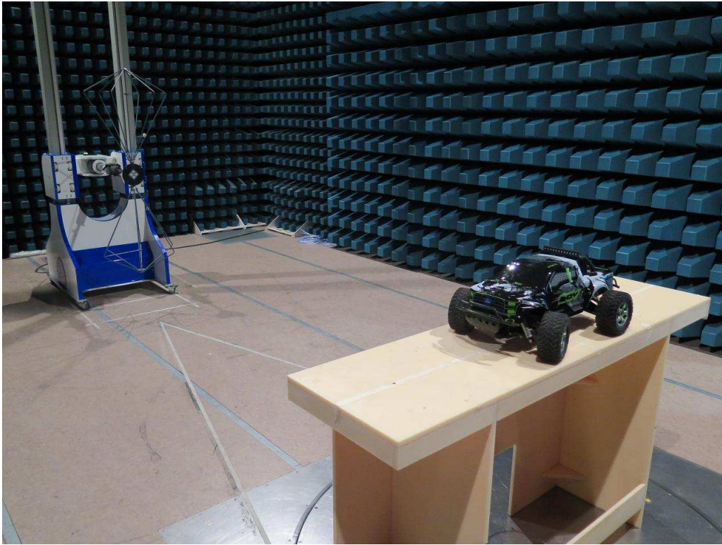
30MHz – 300MHz
