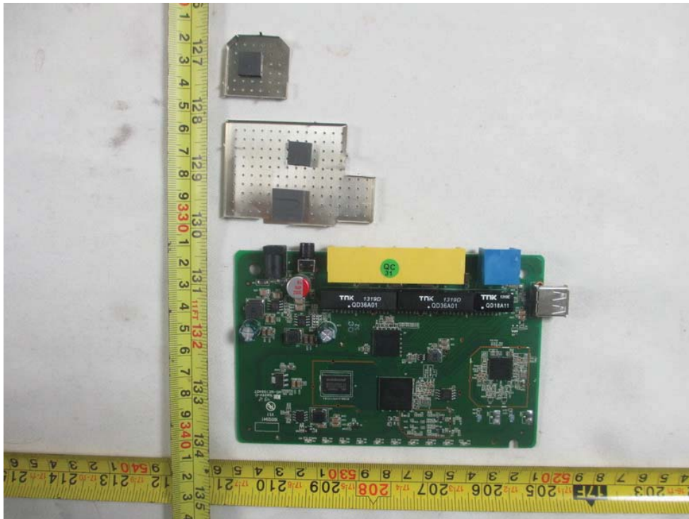
5G RF module IC
