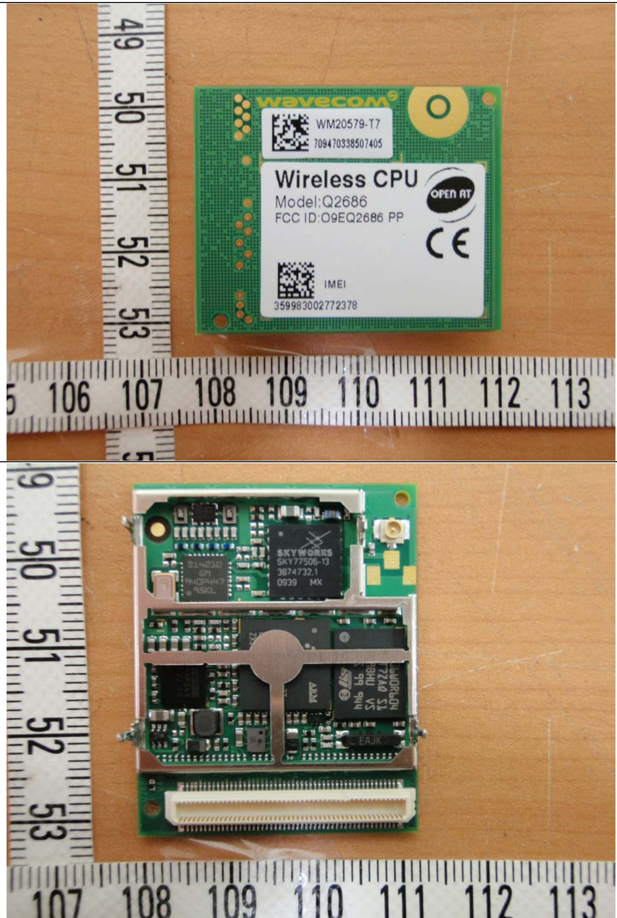
GPRS module
