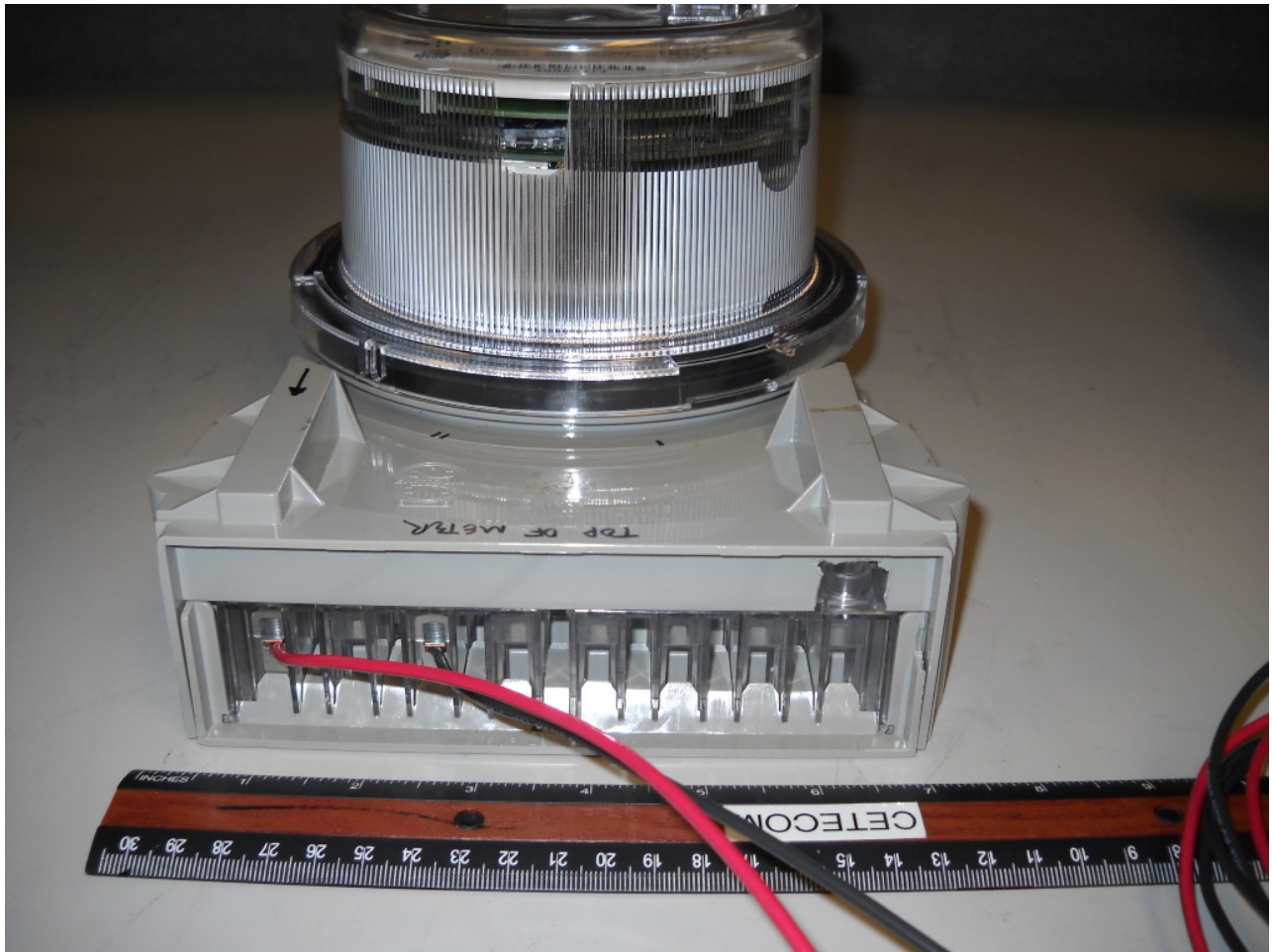
EUT Bottom
