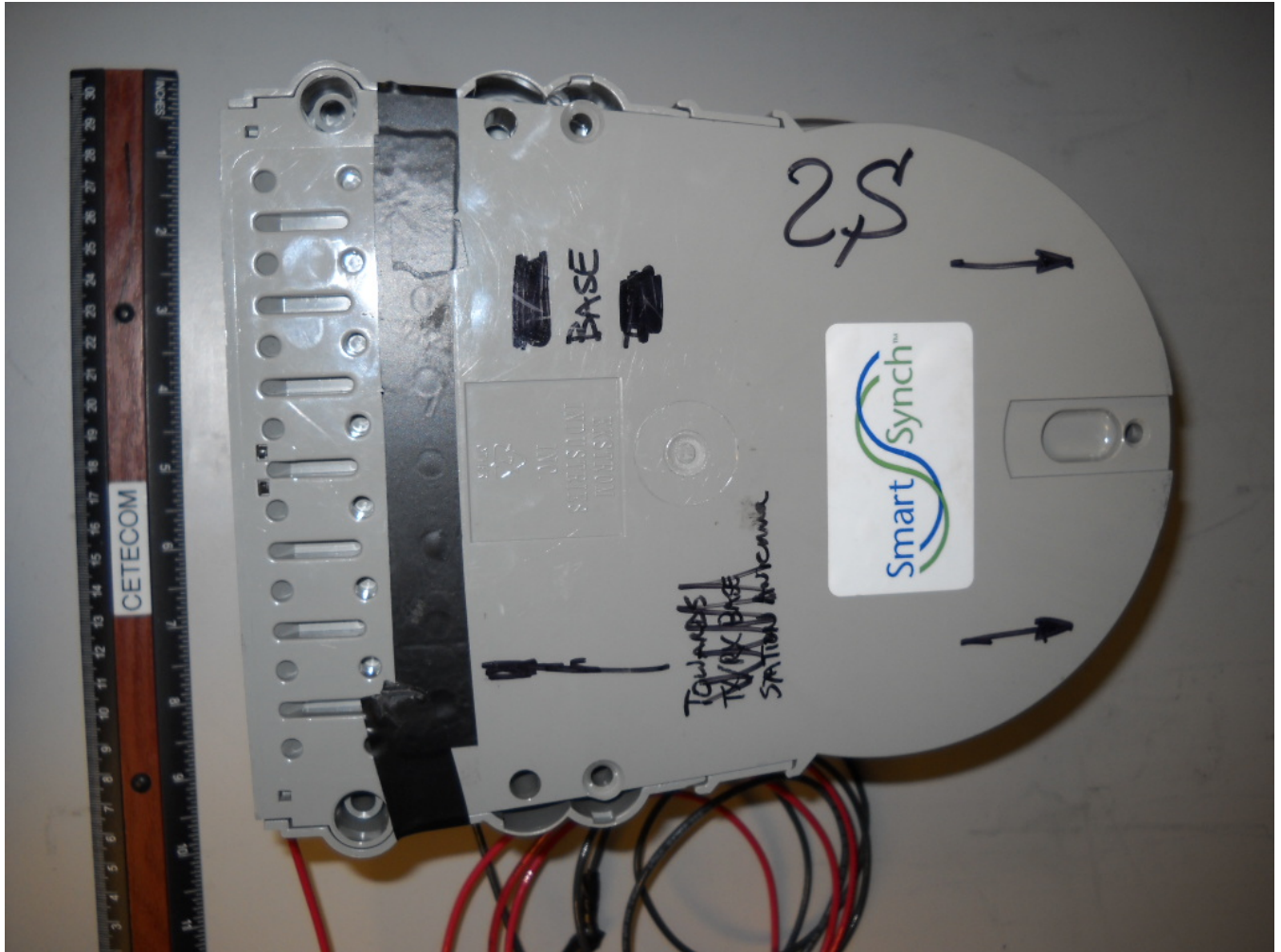
EUT Back
