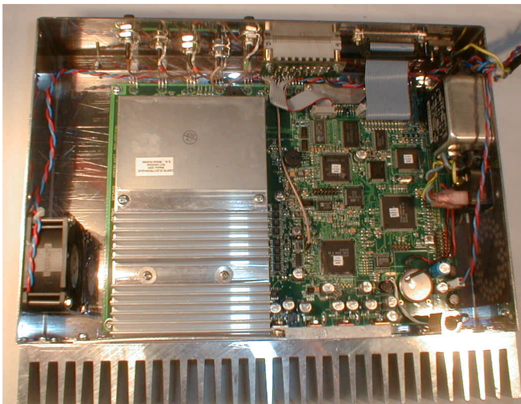
Medio L200 Inside
