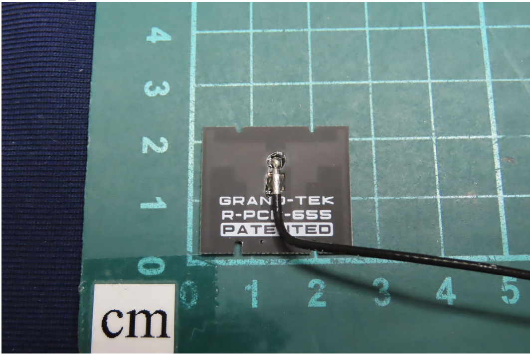
(20) EUT Photo_(Antenna)
