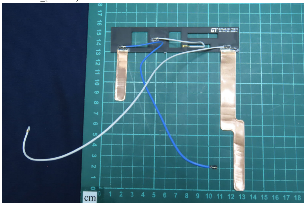
(24) EUT Photo_(Antenna)
