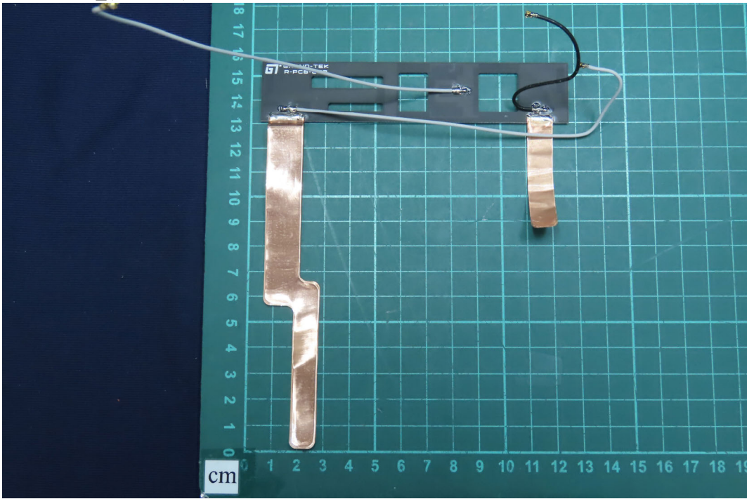
(26) EUT Photo_(Antenna)
