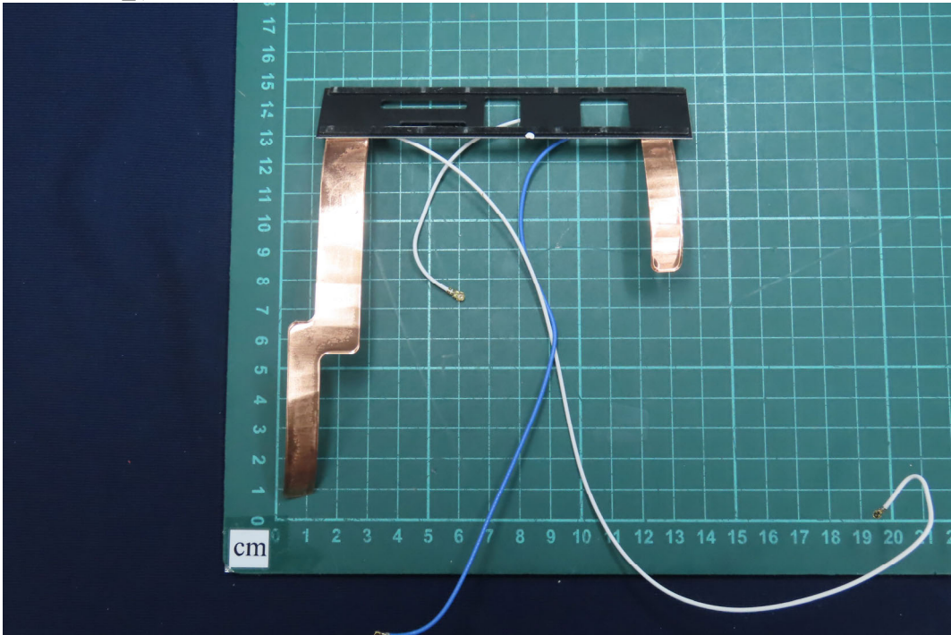
(25) EUT Photo_(Antenna)
