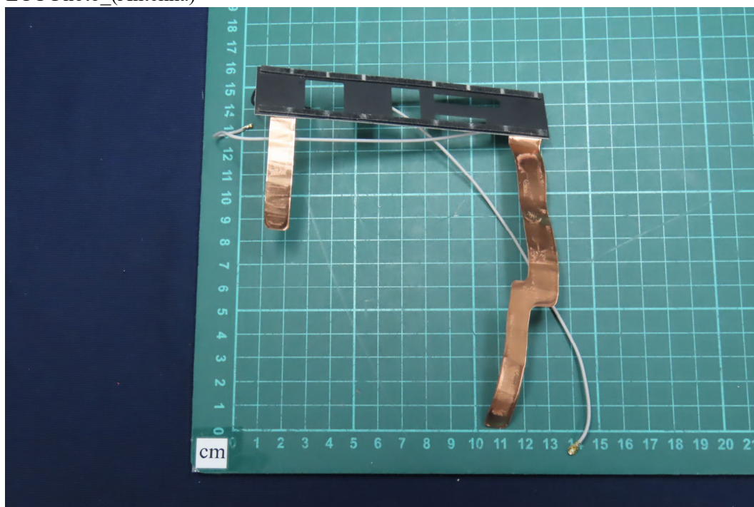
(27) EUT Photo_(Antenna)
