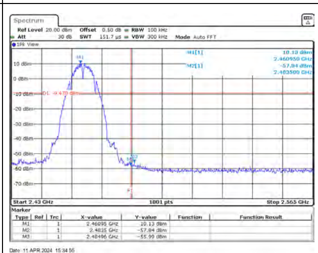
802.11g / 2462 MHz
