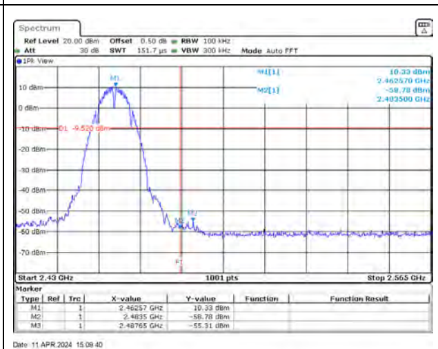
802.11b / 2462 MHz
