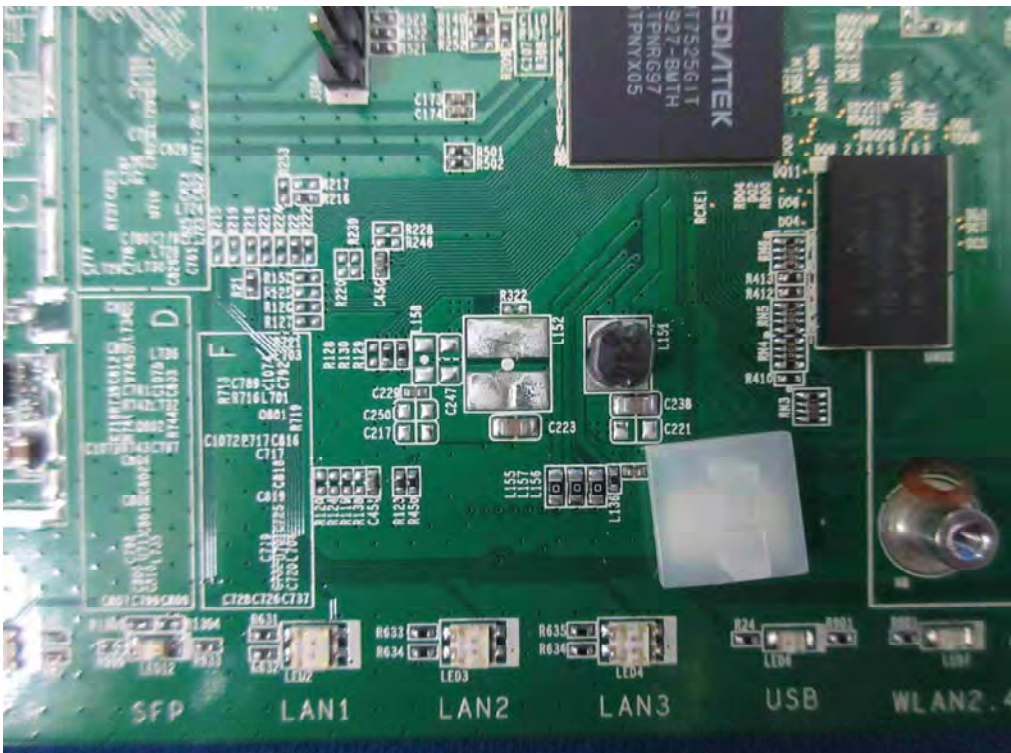
(20) EUT Photo
