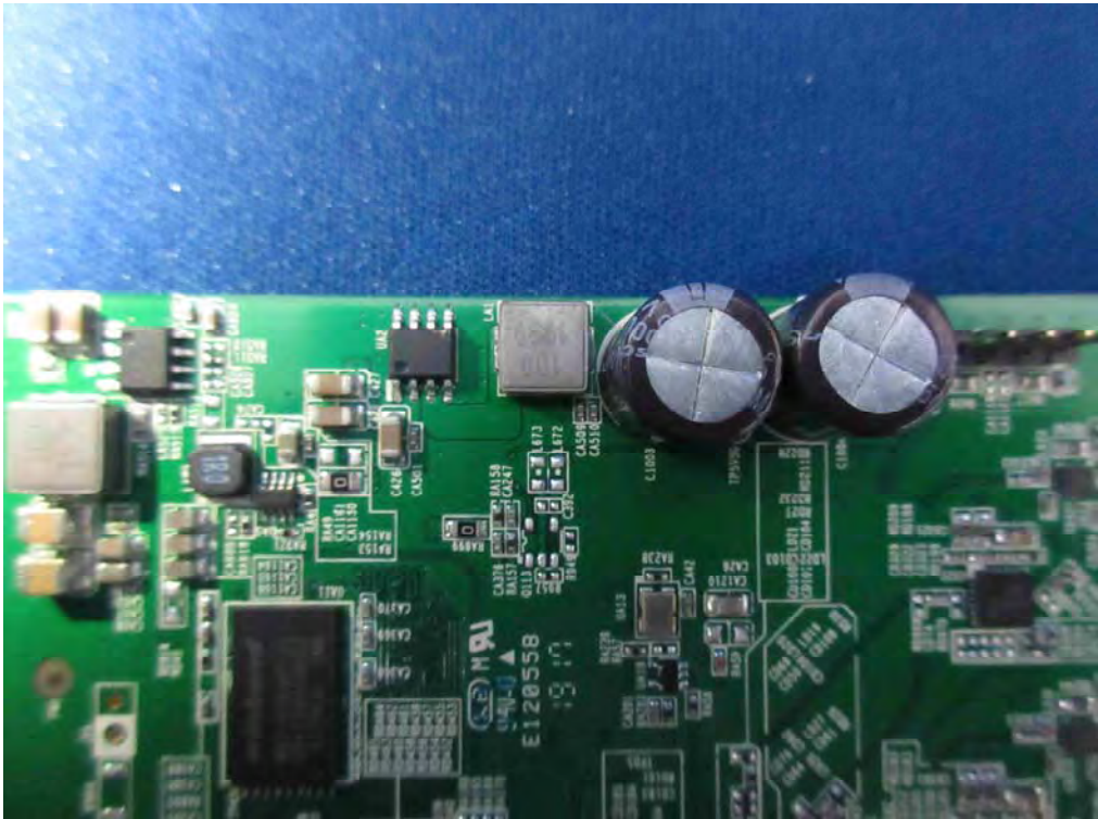
(48) EUT Photo
