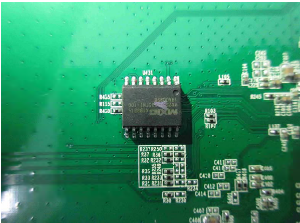
(36) EUT Photo
