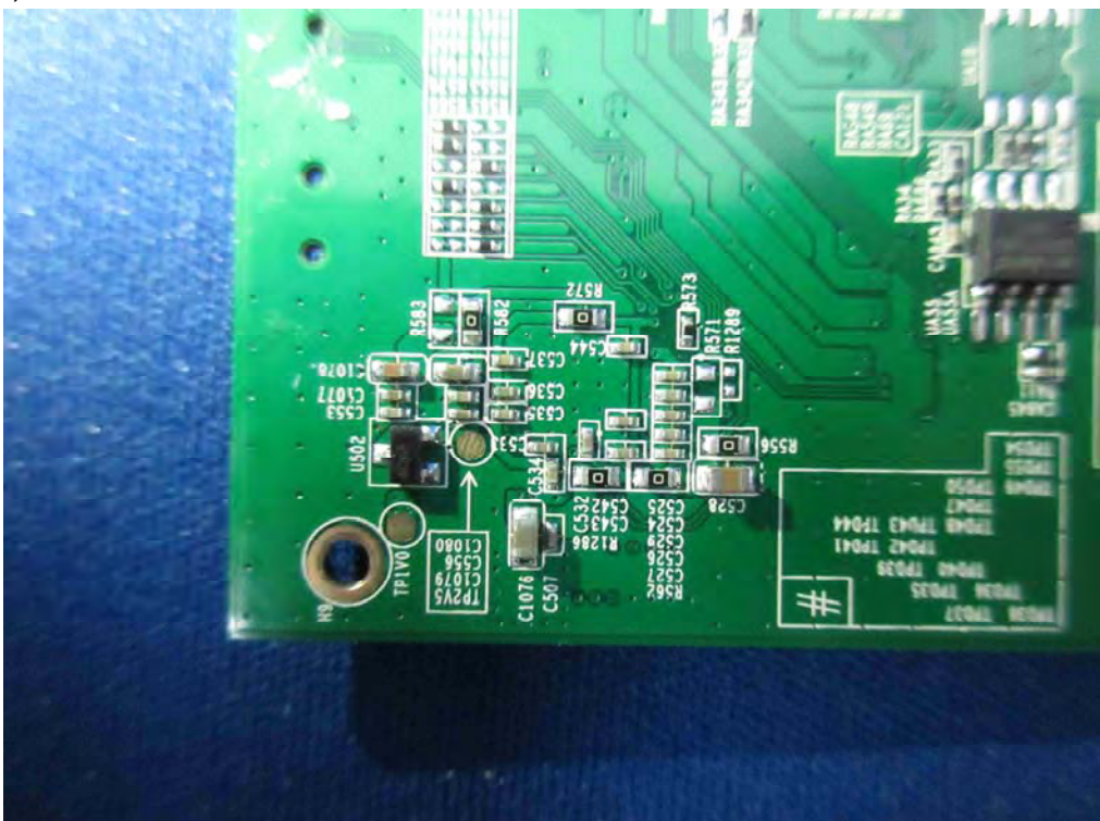
(46) EUT Photo
