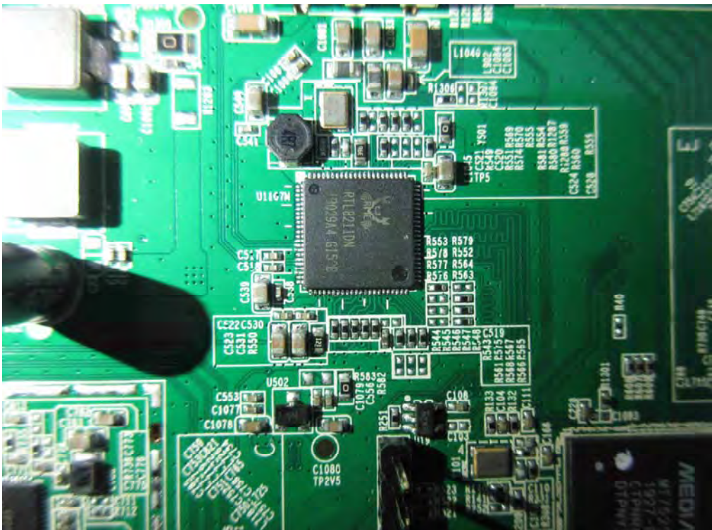
(18) EUT Photo
