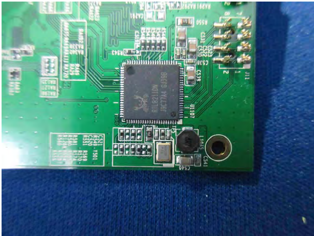
(60) EUT Photo
