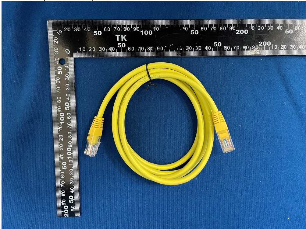
(10) EUT Photo (RJ-45 Cable)
