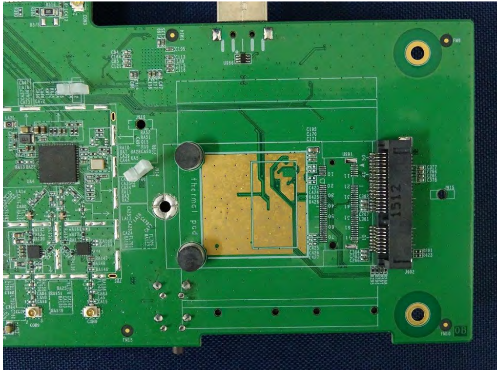
(19) EUT Photo
