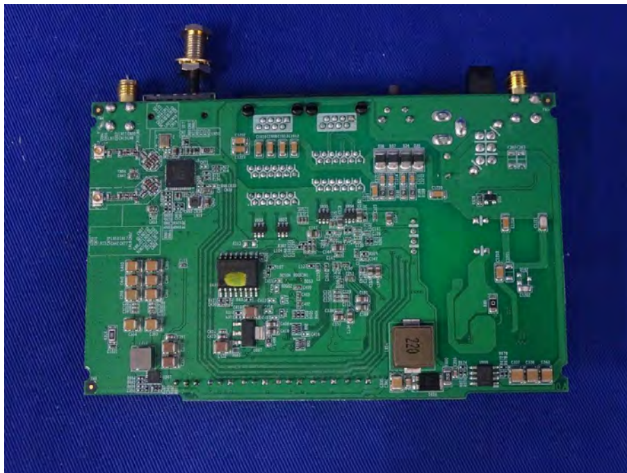
(12) EUT Photo WLAN Module
