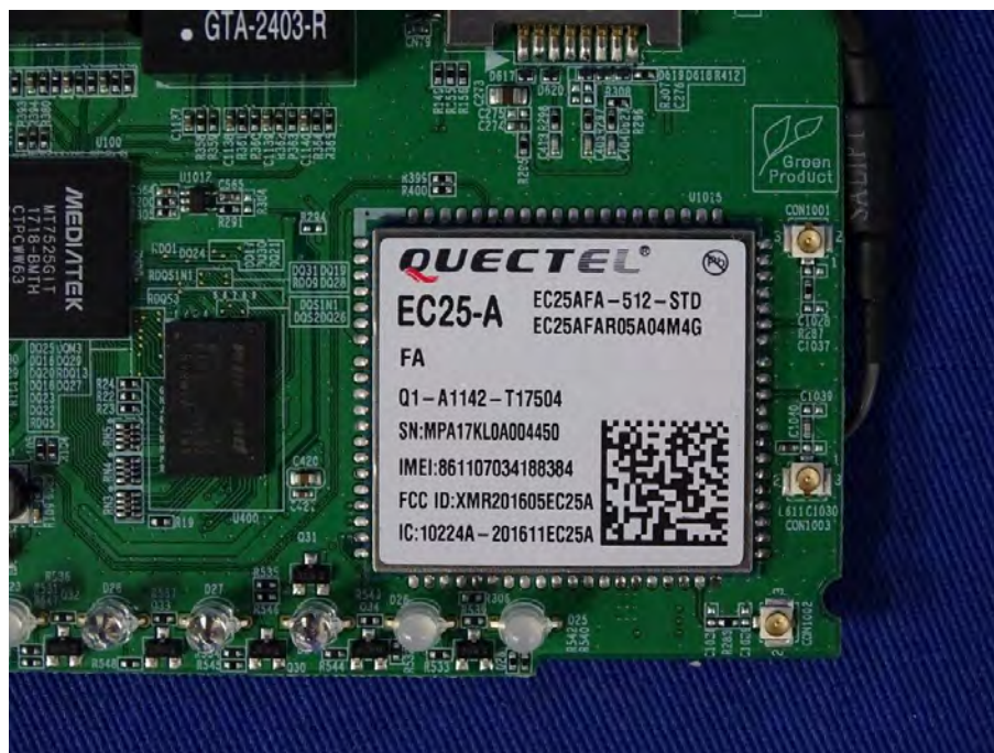
(16) EUT Photo WWAN Module
