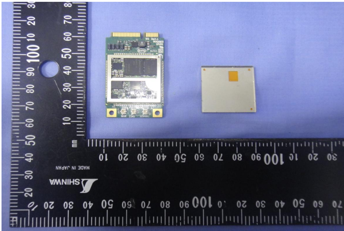
RF IC
