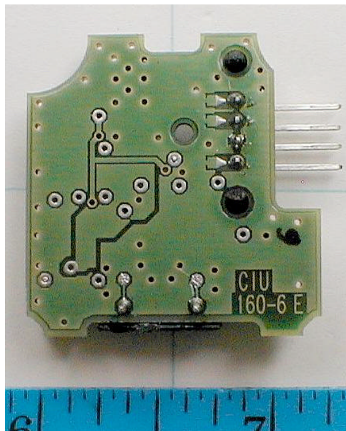
PCB Bottom
