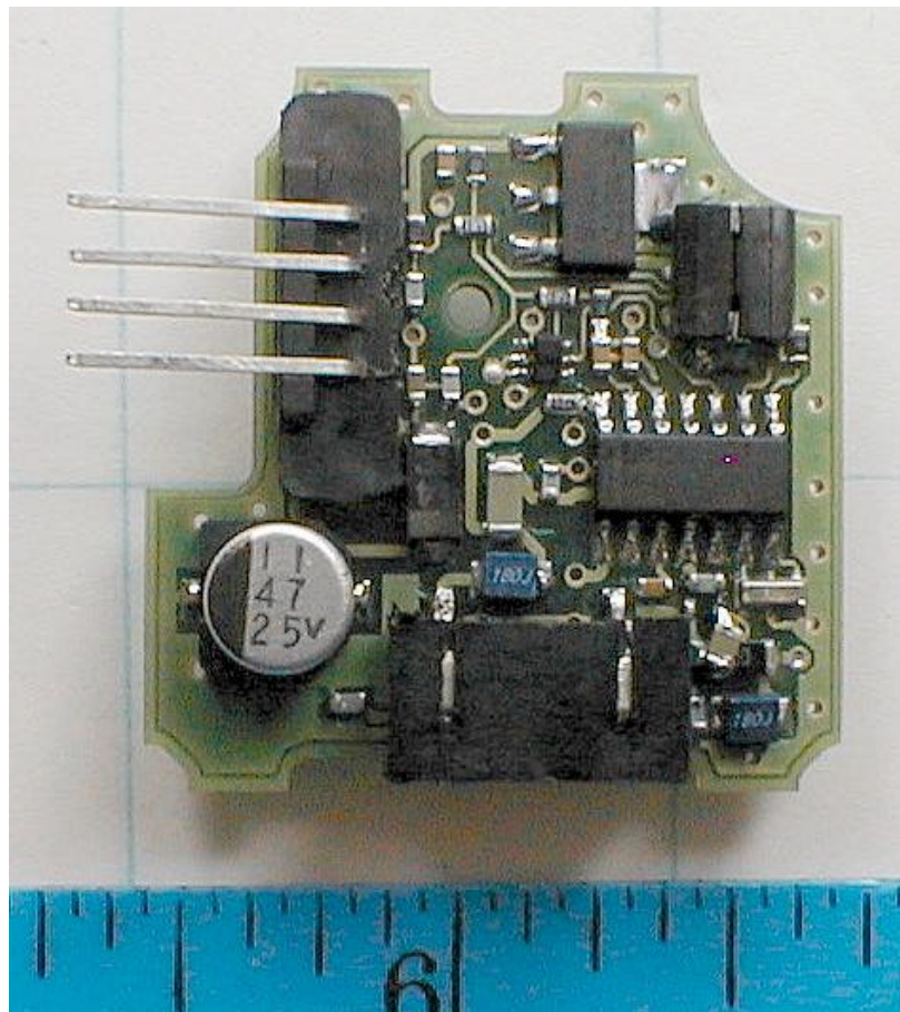
PCB Top
