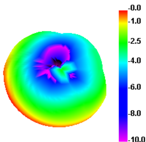
2450.000MHz E1
