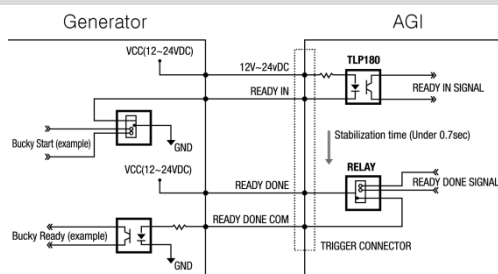
&lt;Assembly Diagram&gt;
