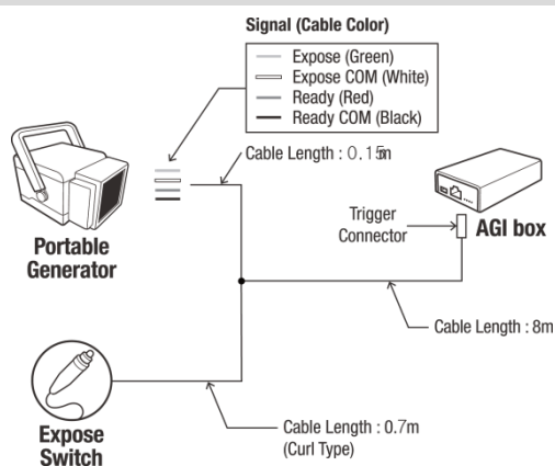
&lt;Assembly Diagram&gt;
