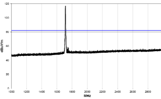
WCDMA – 1712.4MHz
