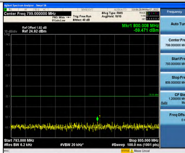
Band13-Stand-Alone-NaB-BPSK-23230-1@11-15kHz-793-805-793-805MHz@-59.47dBm--35-PASS
