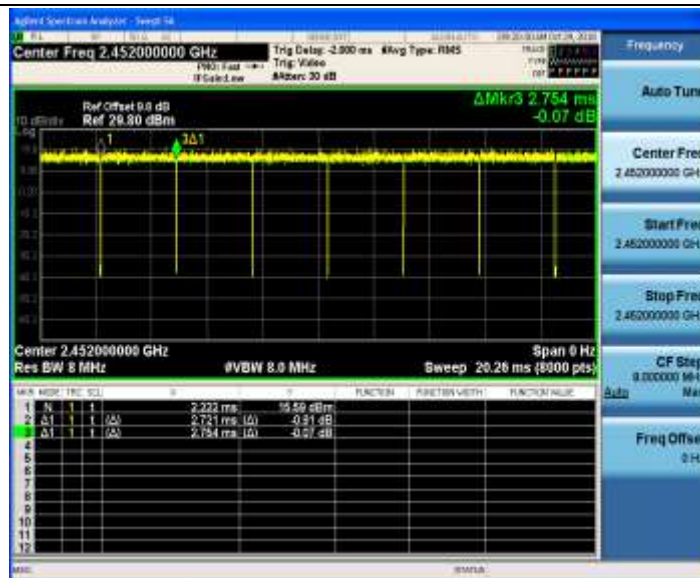
11G-CDD_Ant2_2452
