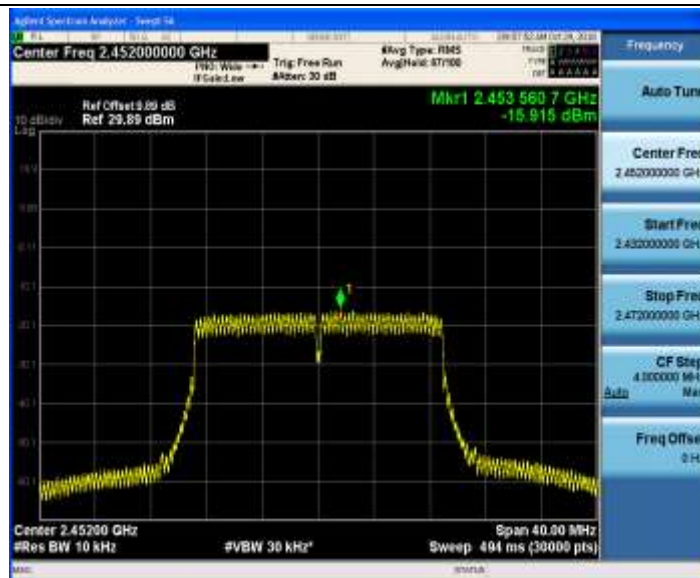
11N20MIMO_Ant2_2452
