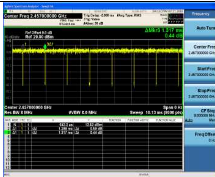
11N20MIMO_Ant2_2457
