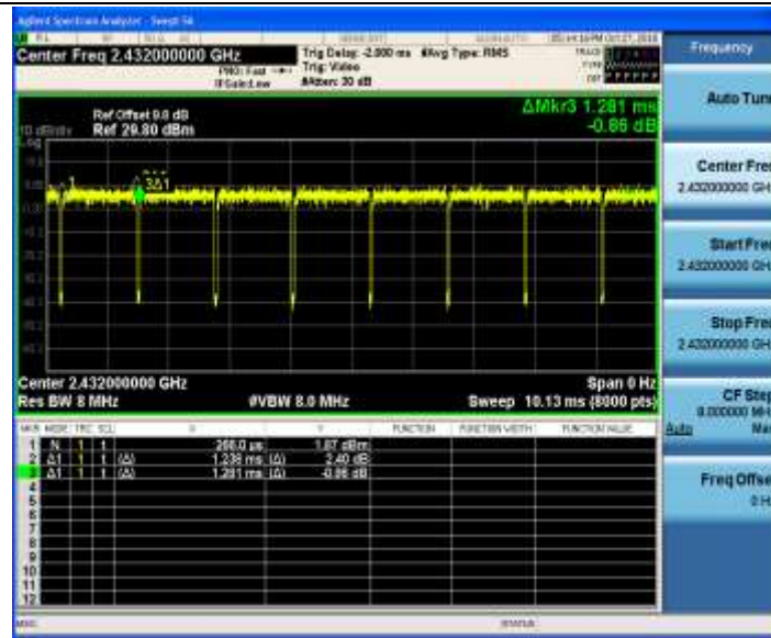
11N40SISO_Ant2_2432
