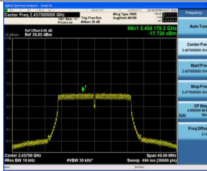
11N20SISO_Ant2_2457
