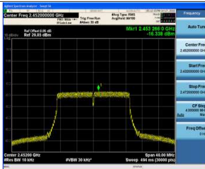
11N20SISO_Ant2_2452
