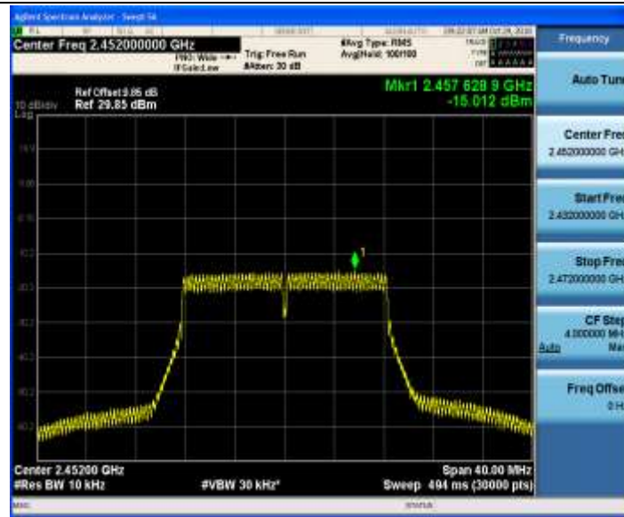
11G-CDD_Ant2_2452
