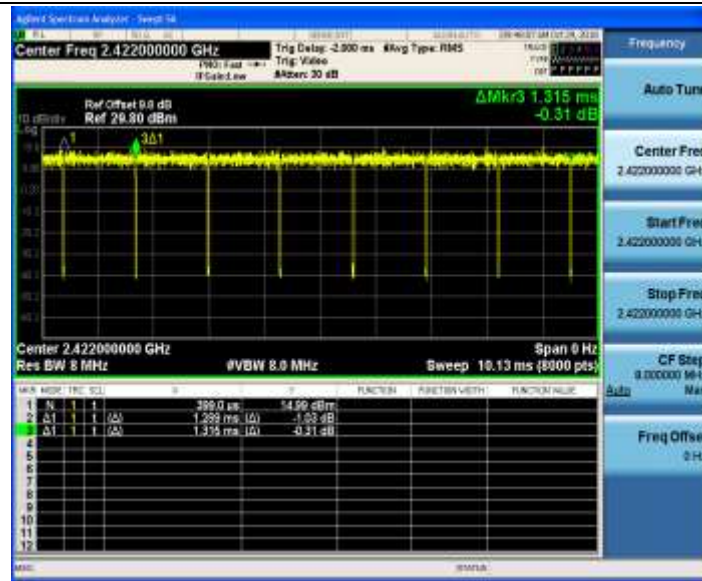
11N20MIMO_Ant2_2422
