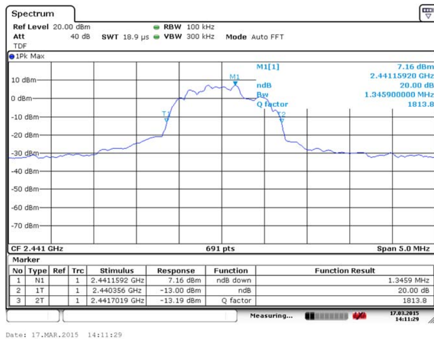
Fig. 87 Occupied 20dB Bandwidth ( \pi/4 DQPSK, Ch 39)
