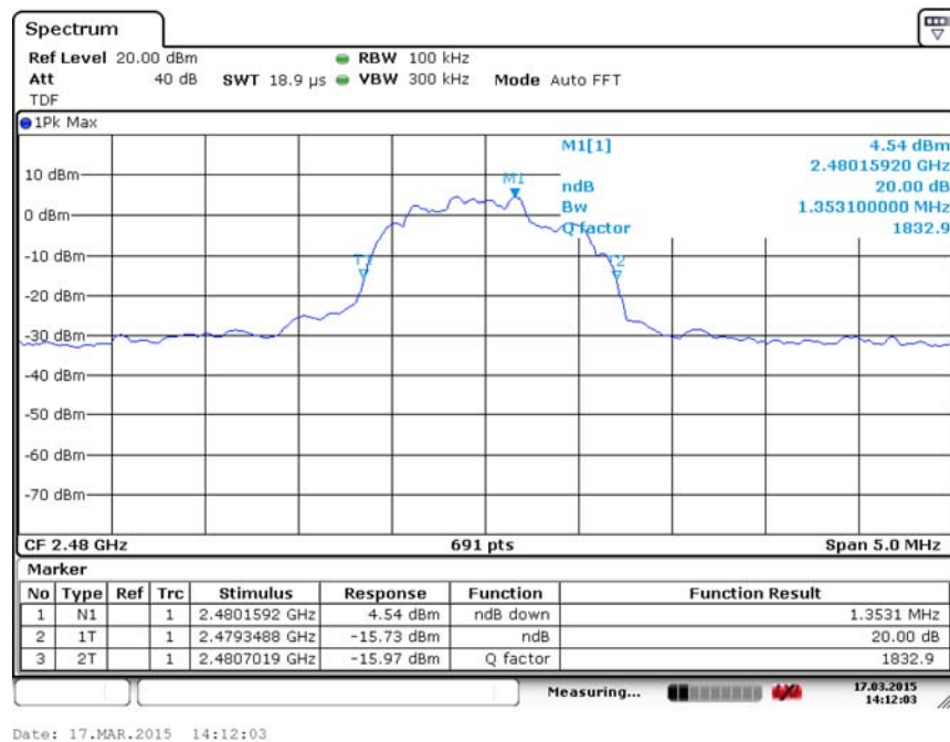
Fig. 88 Occupied 20dB Bandwidth ( \pi/4 DQPSK, Ch 78)
