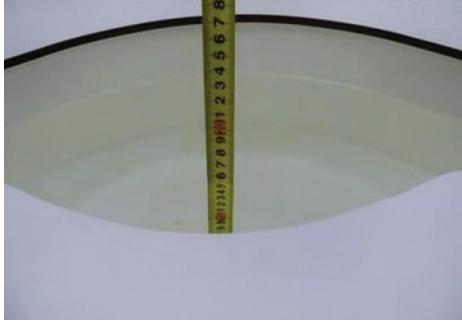
Body 2450 MHz 15.4cm
