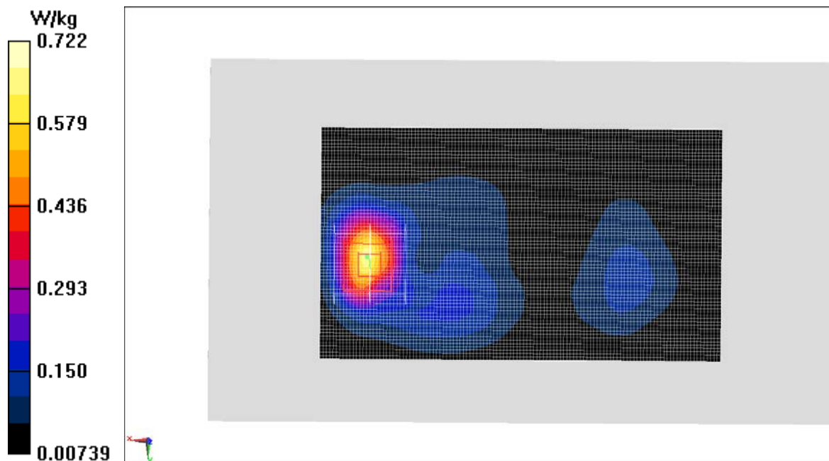
Fig.6 WCDMA1900
