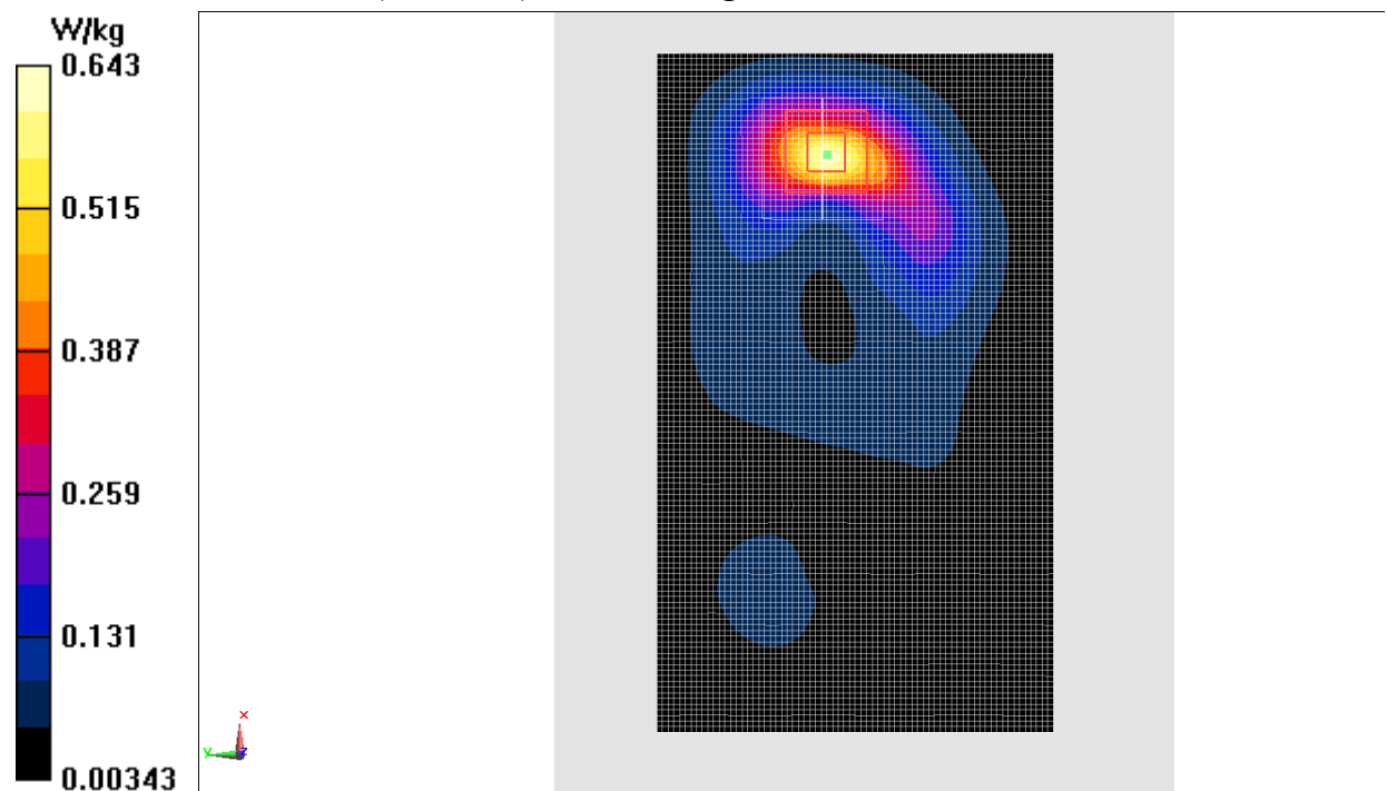
Fig.9 LTE Band7
