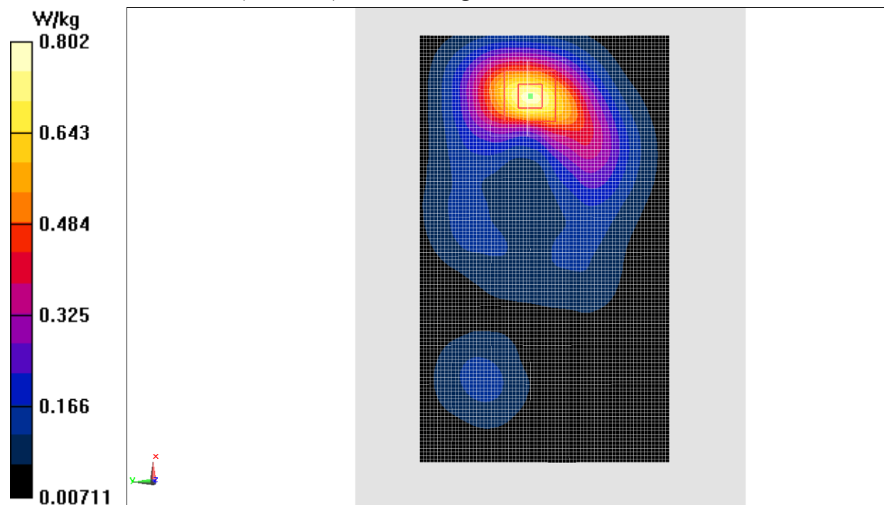
Fig.8 LTE Band7
