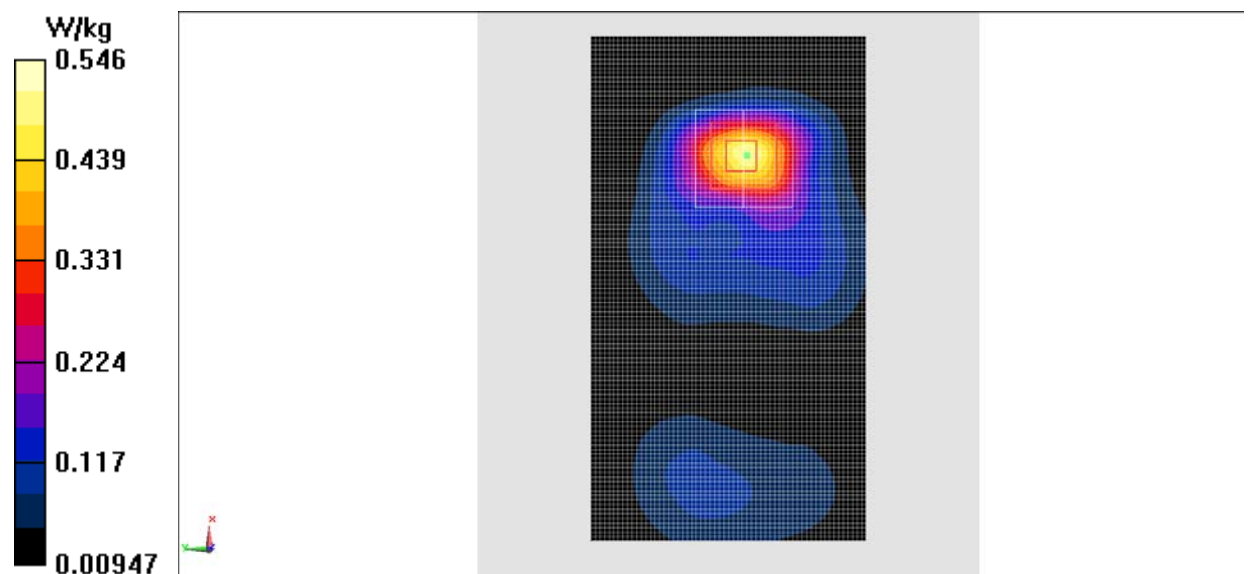
Fig.16 LTE Band4
