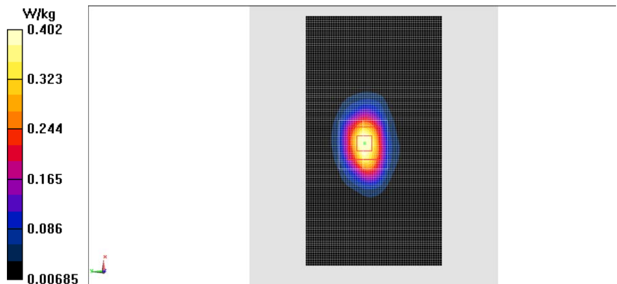
Fig.9 WCDMA1700
