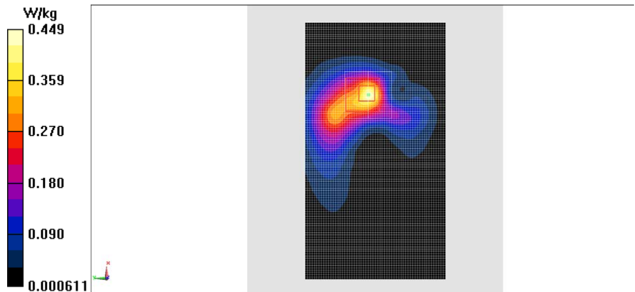
Fig.19 LTE Band7
