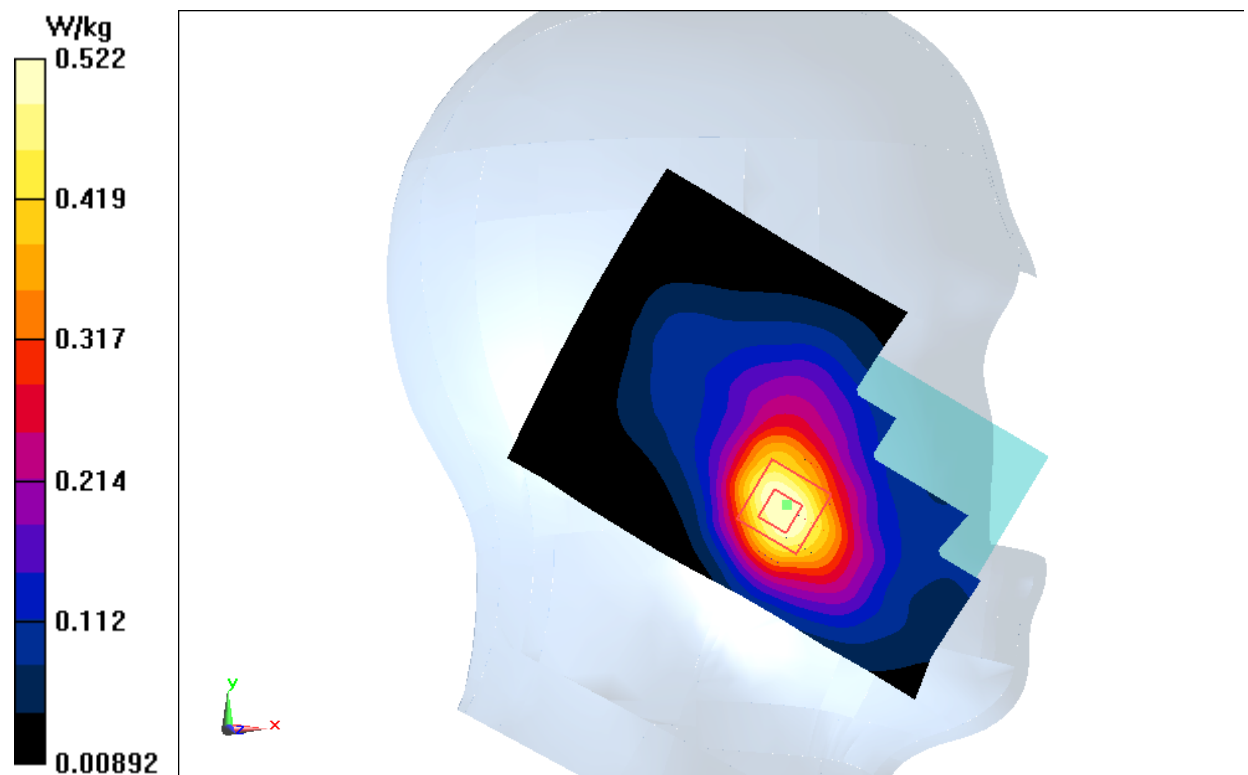
Fig.7 WCDMA1700
