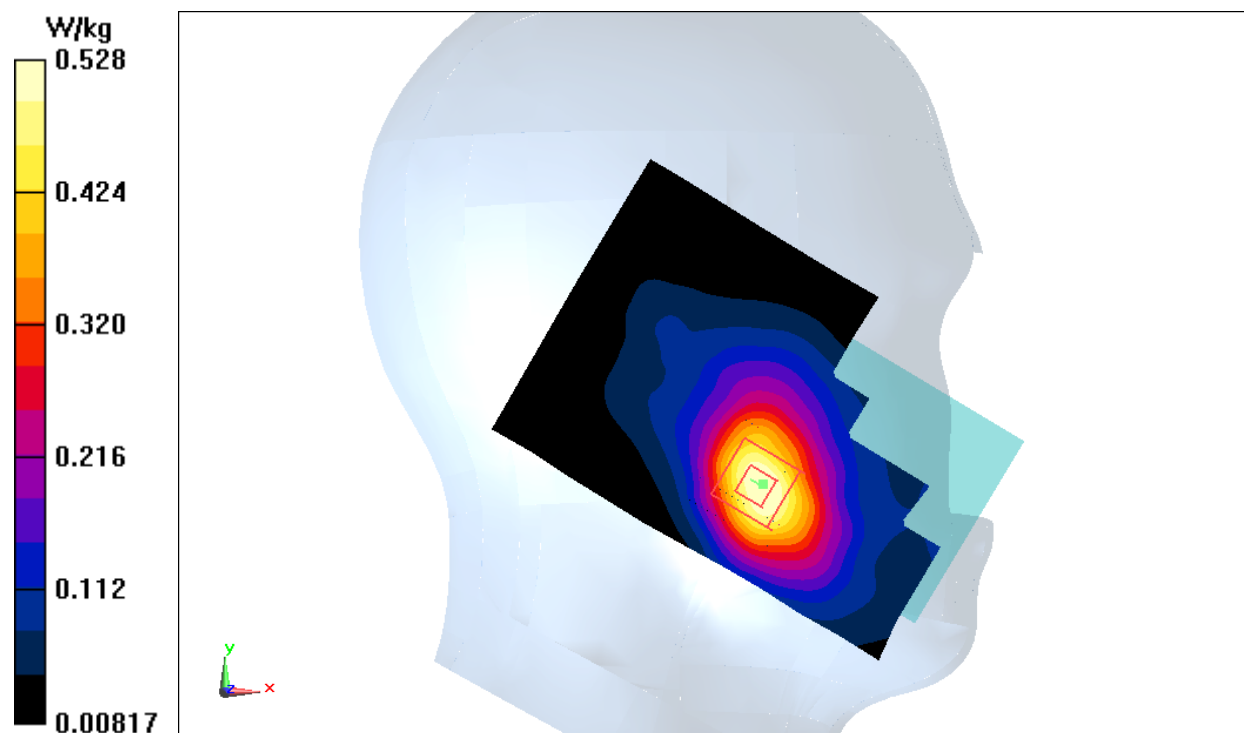
Fig.14 LTE Band4
