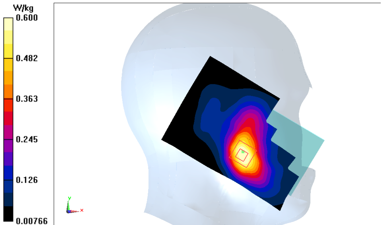
Fig.12 LTE Band2
