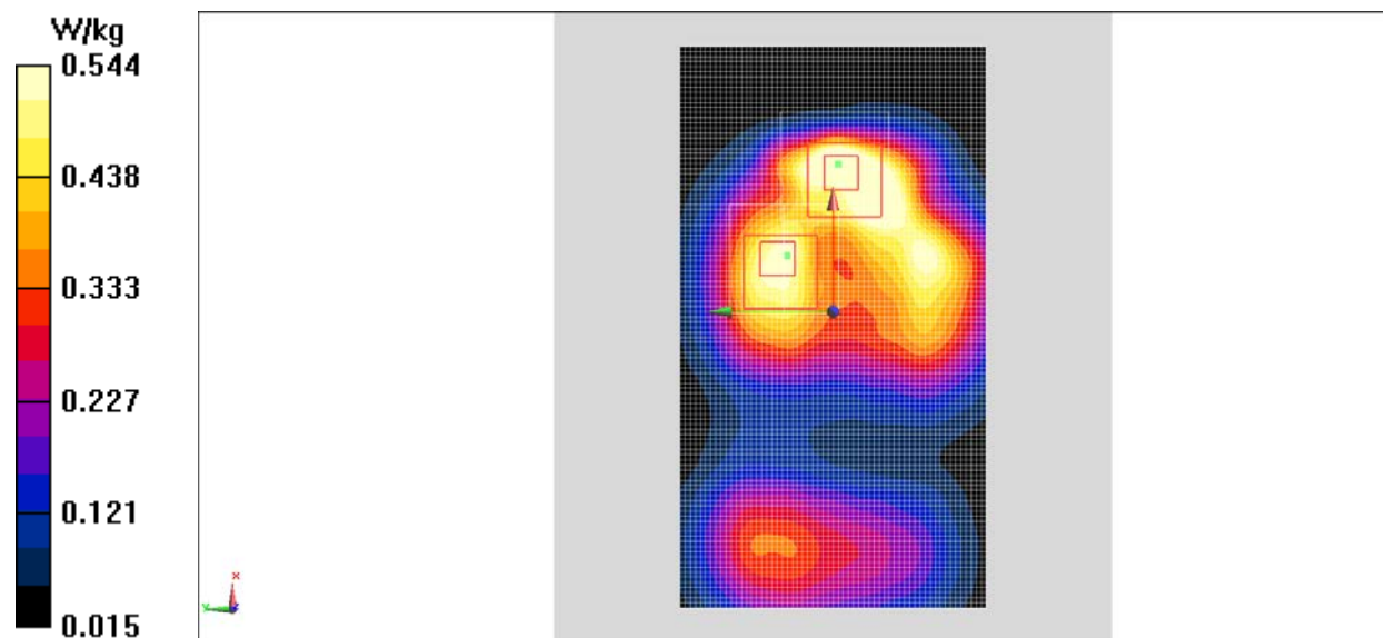
Fig.13 LTE Band2
