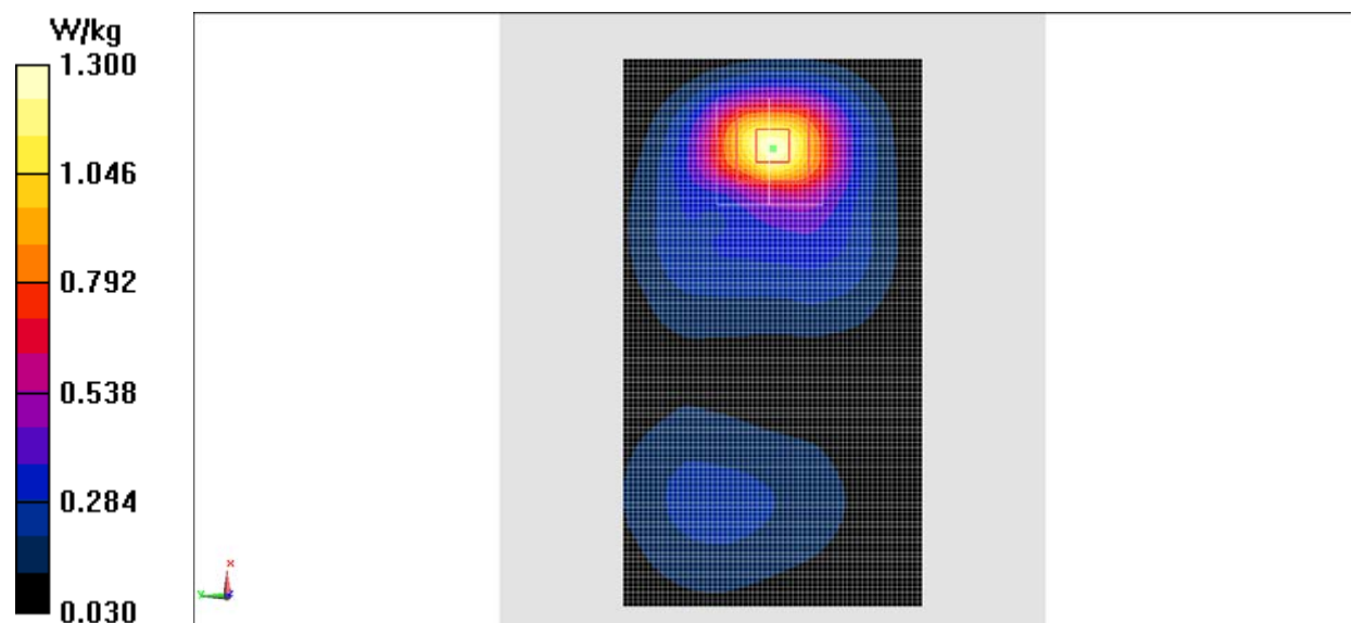
Fig.8 WCDMA1700
