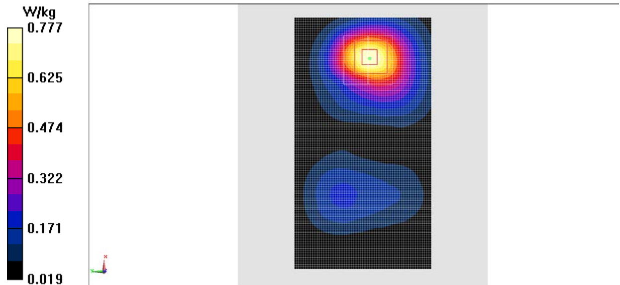
Fig.15 LTE Band4
