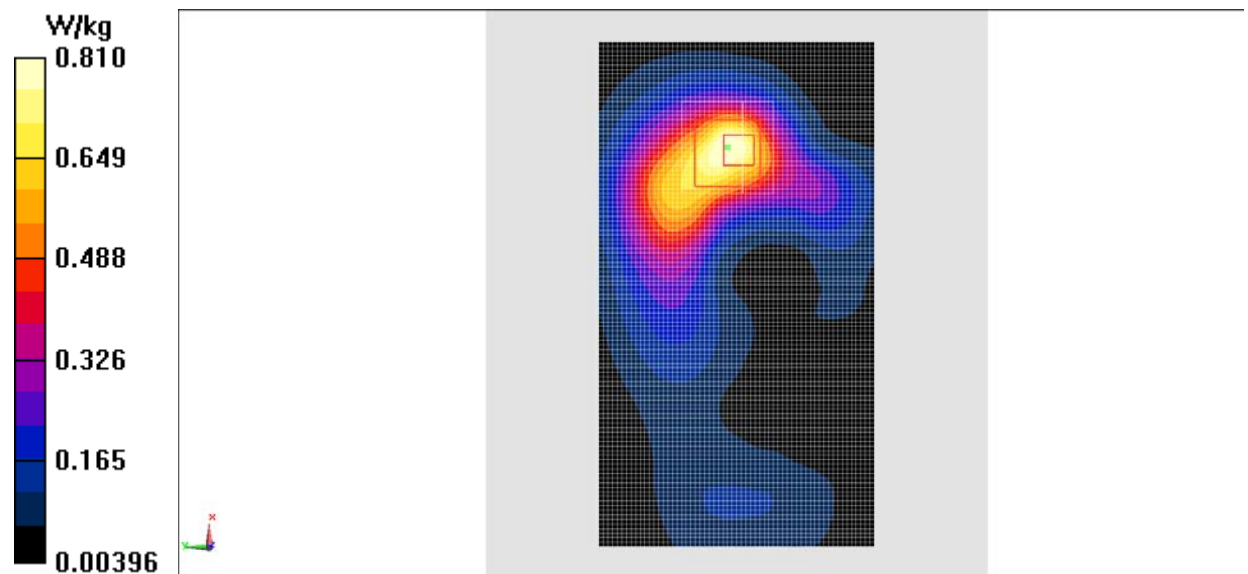
Fig.18 LTE Band7
