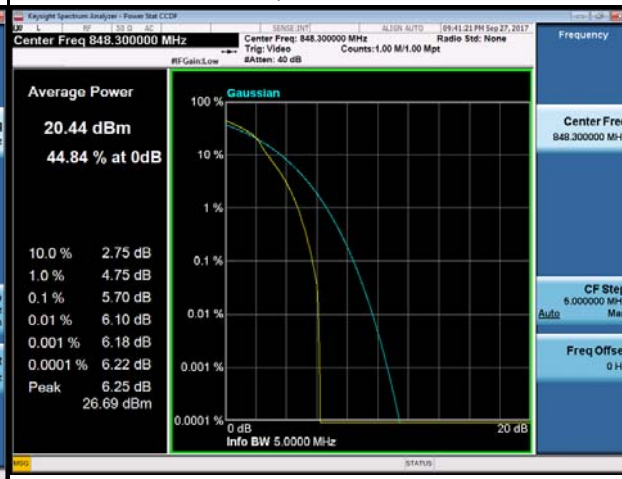
16QAM-27033
