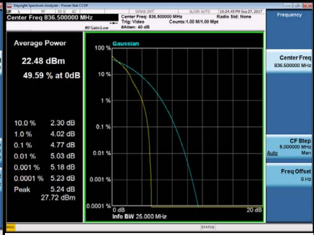
16QAM-26865
