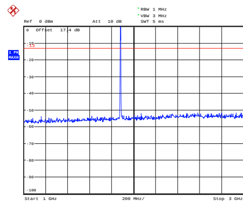
GSM 1900 CH-Middle 1GHz~3GHz
