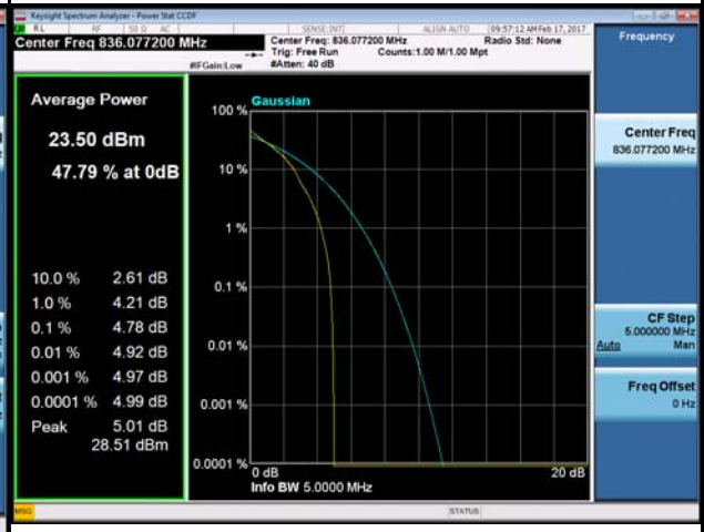
16QAM-20407
