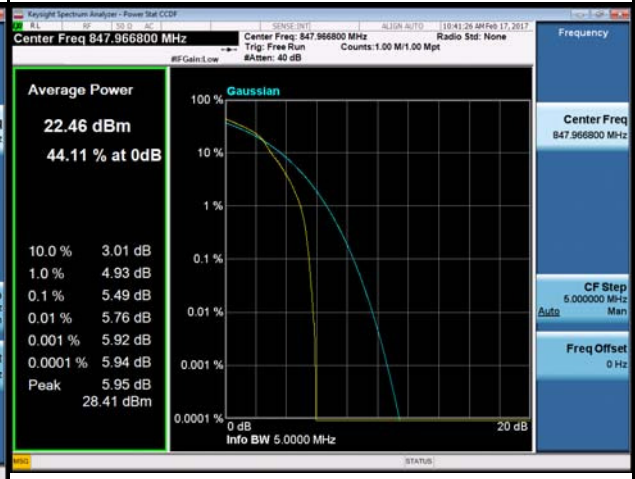
16QAM-20643
