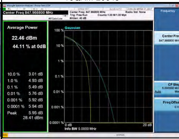
16QAM-20643
