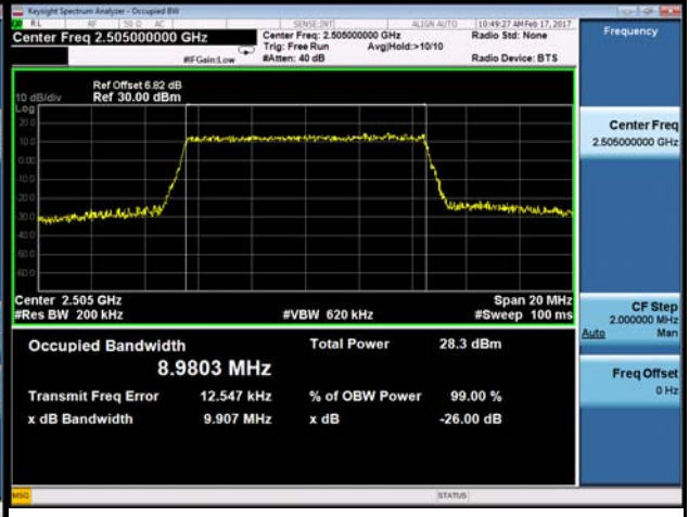
16QAM-21400
