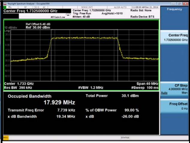
16QAM-20050
