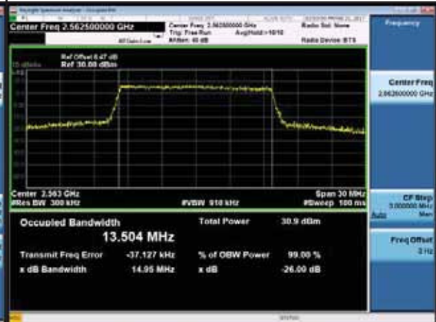
16QAM-21375
