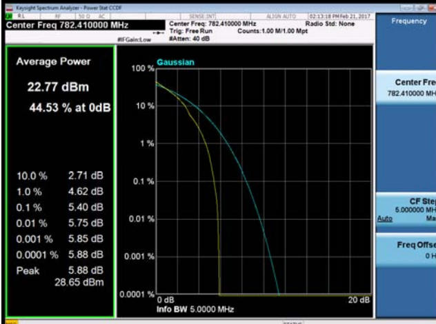
16QAM-23230
