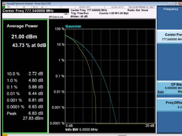
QPSK-23255
