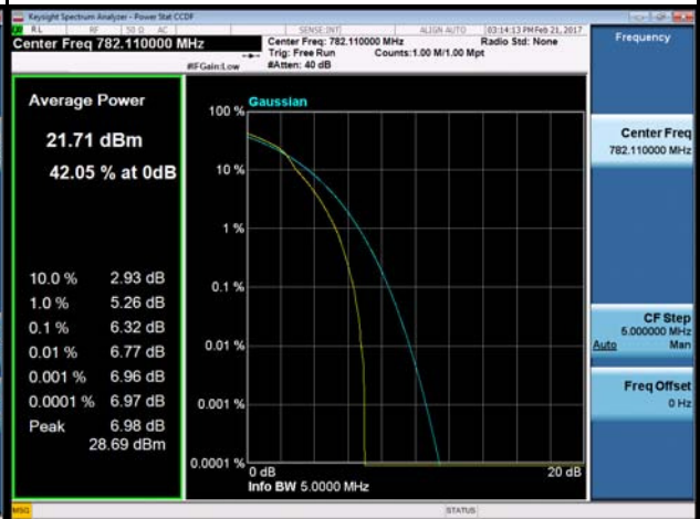
16QAM-23255
