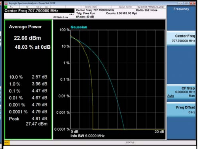
16QAM-23755
