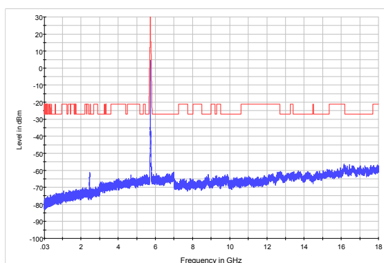
Frequency 5735MHz, 30M-18GHz
