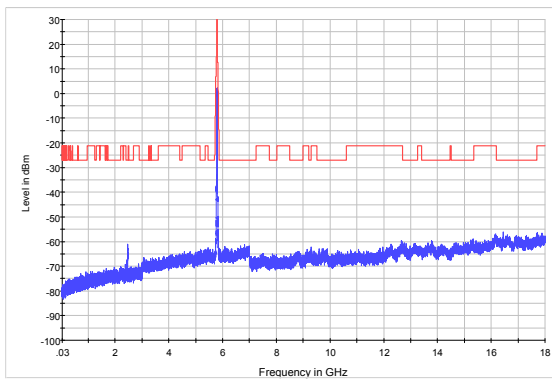
Frequency 5790MHz, 30M-18GHz
