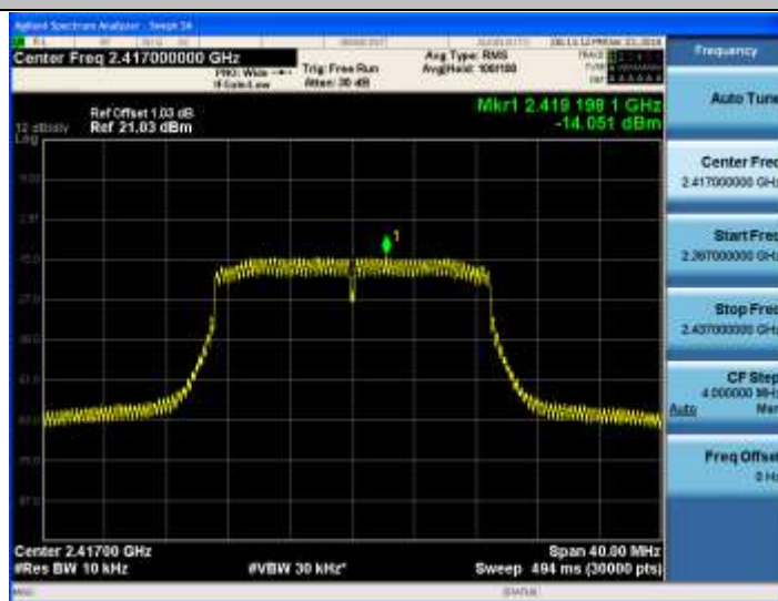
11N20SISO_Ant2_2417
