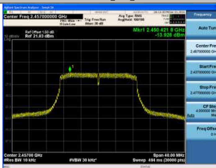
11N20SISO_Ant2_2457
