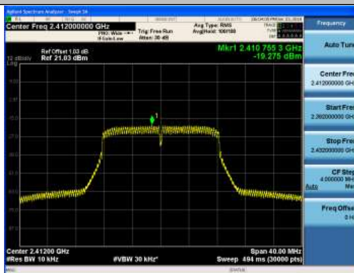
11G-CDD_Ant2_2412
