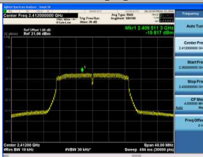
11N20MIMO_Ant2_2412
