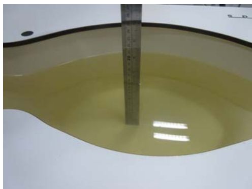
Body(1750MHz)_16.00cm
