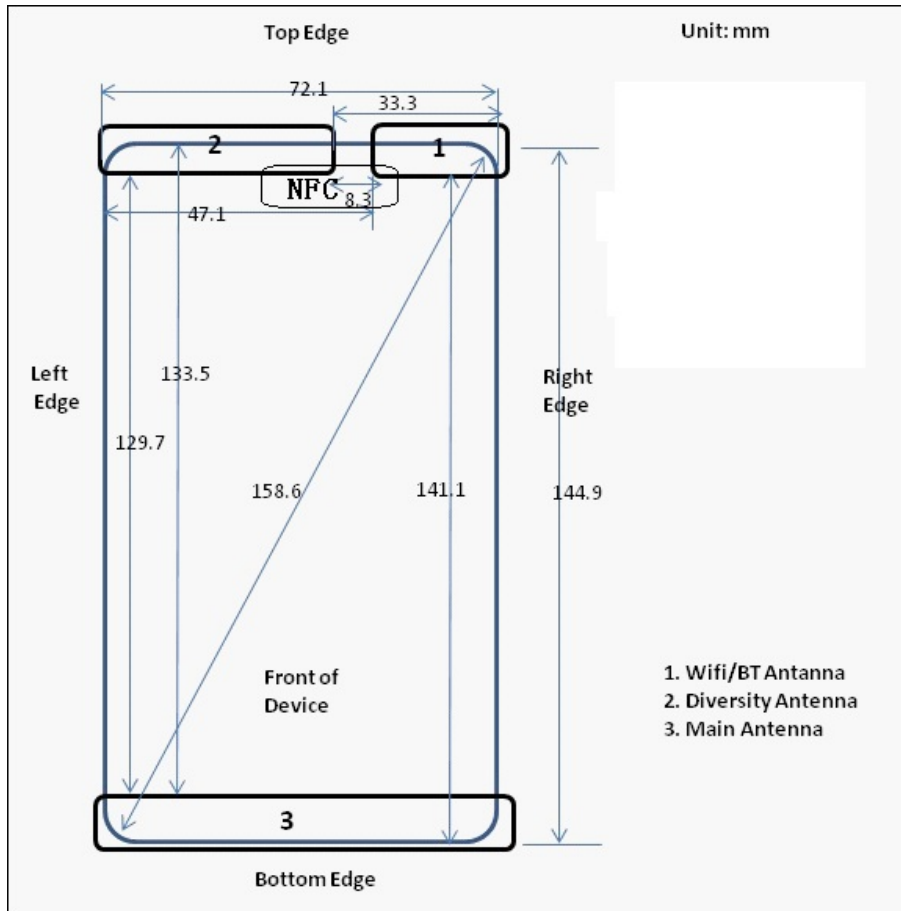
b: Antenna
