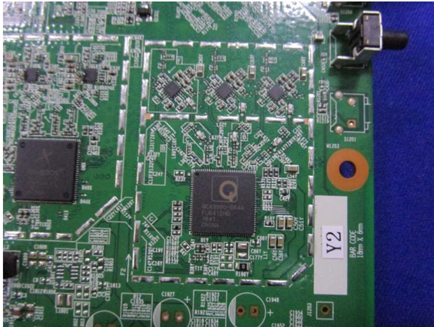
EUT – 5G Module View
