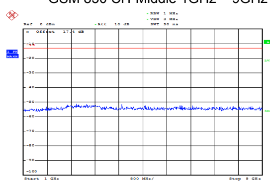
GSM 850 CH-Middle 1GHz ~ 9GHz
