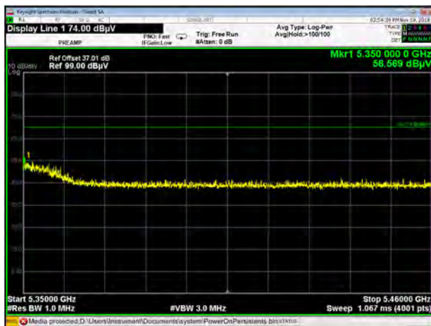
Band II 11n40 CH62
