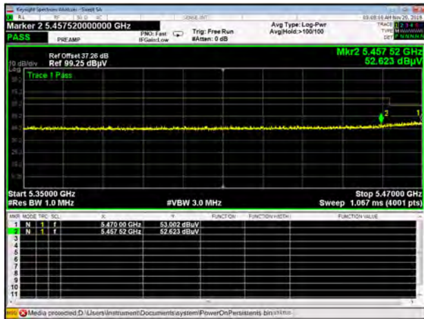
Band III 11n40 CH102
