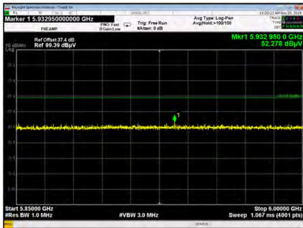
Band III 11n40 CH142
