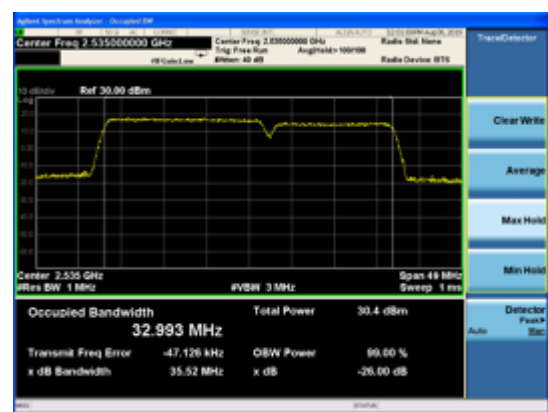
CA-7C QPSK 20MHz+15MHz
