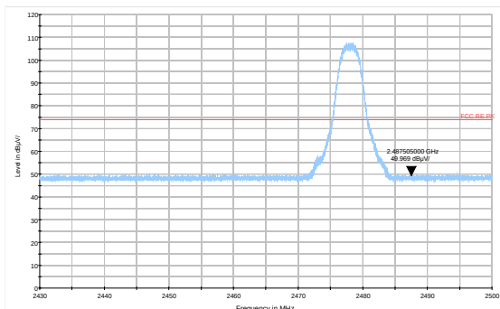
BT 2MHz \pi/4 -DQPSK(4Mbps) 2478MHz: Peak
